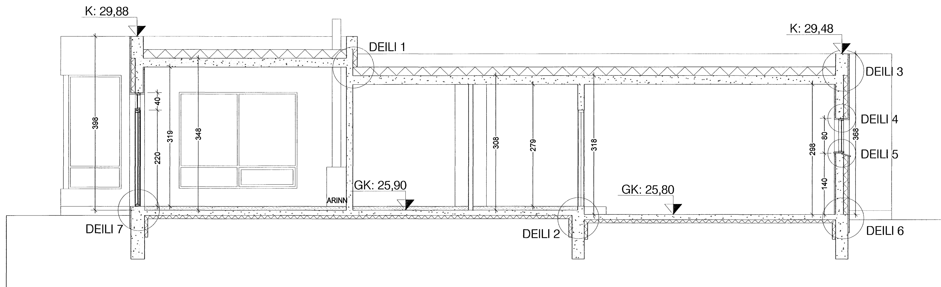
SNEIÐING A-A
