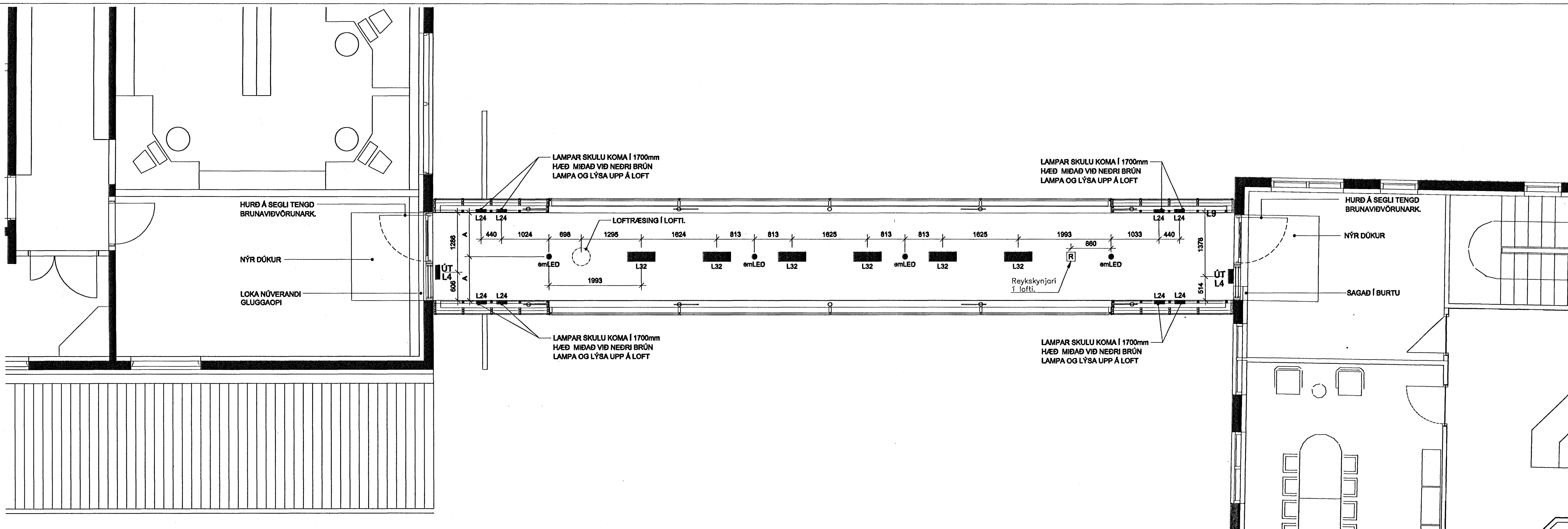
GRUNNMYND 1:50
