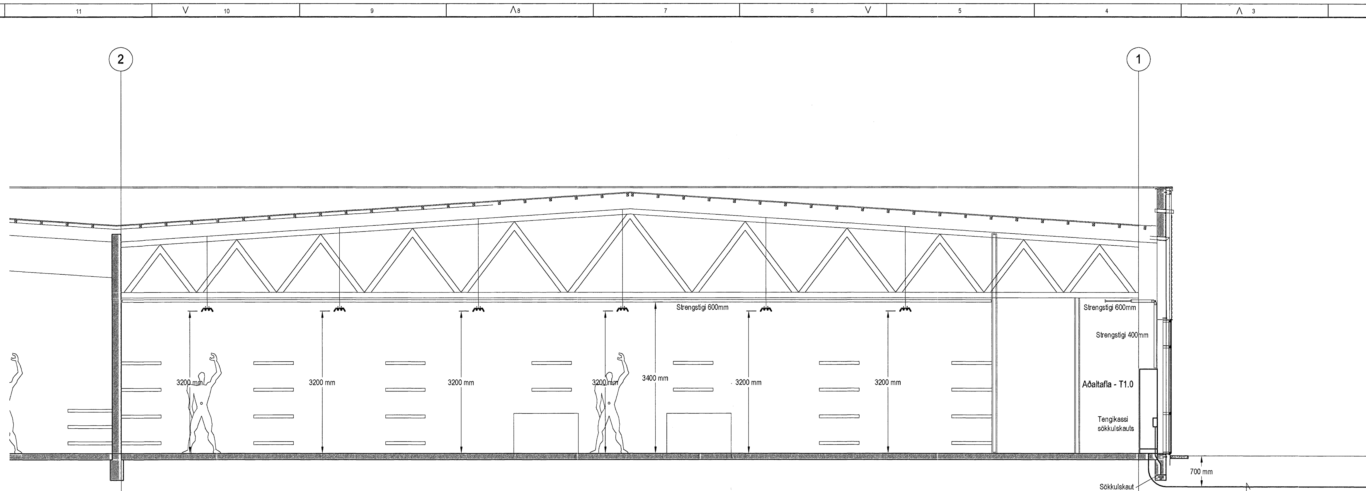
A SNID A Inntakspipur, lampaplan og lagnaleiðir Mkv 1:50
