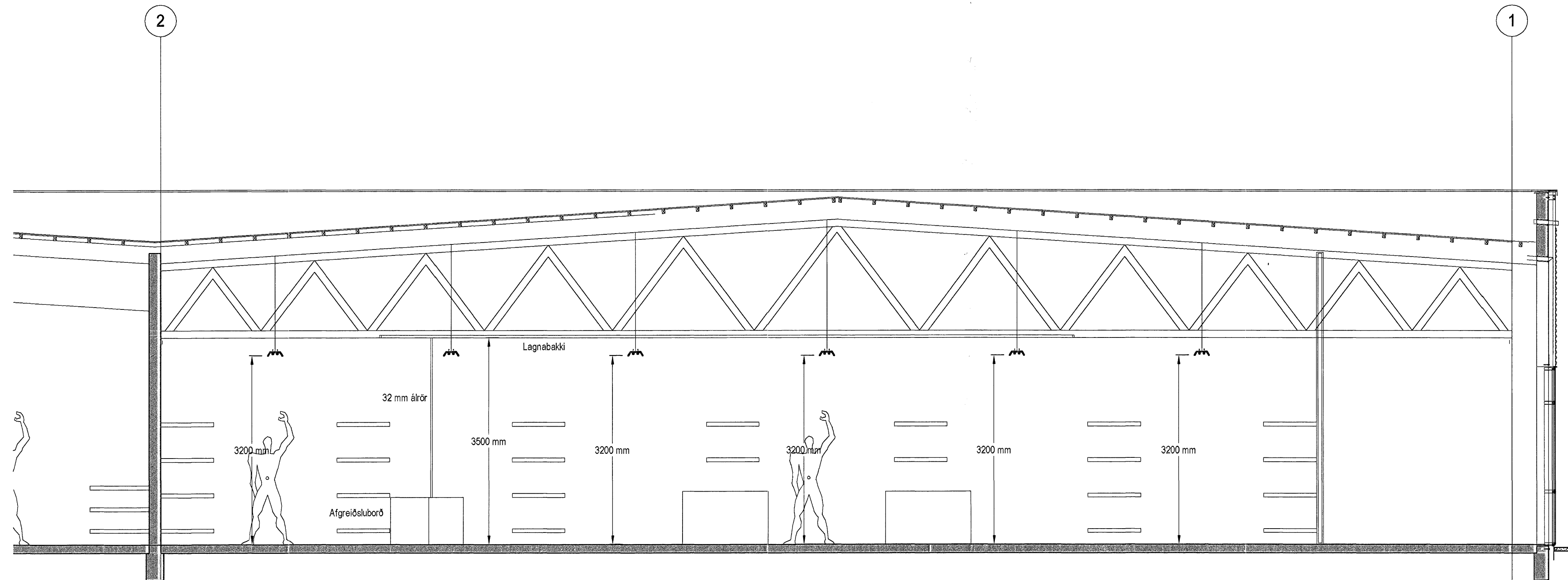
B SNID B Lampaplan og lagnaleiðir Mkv 1:50
