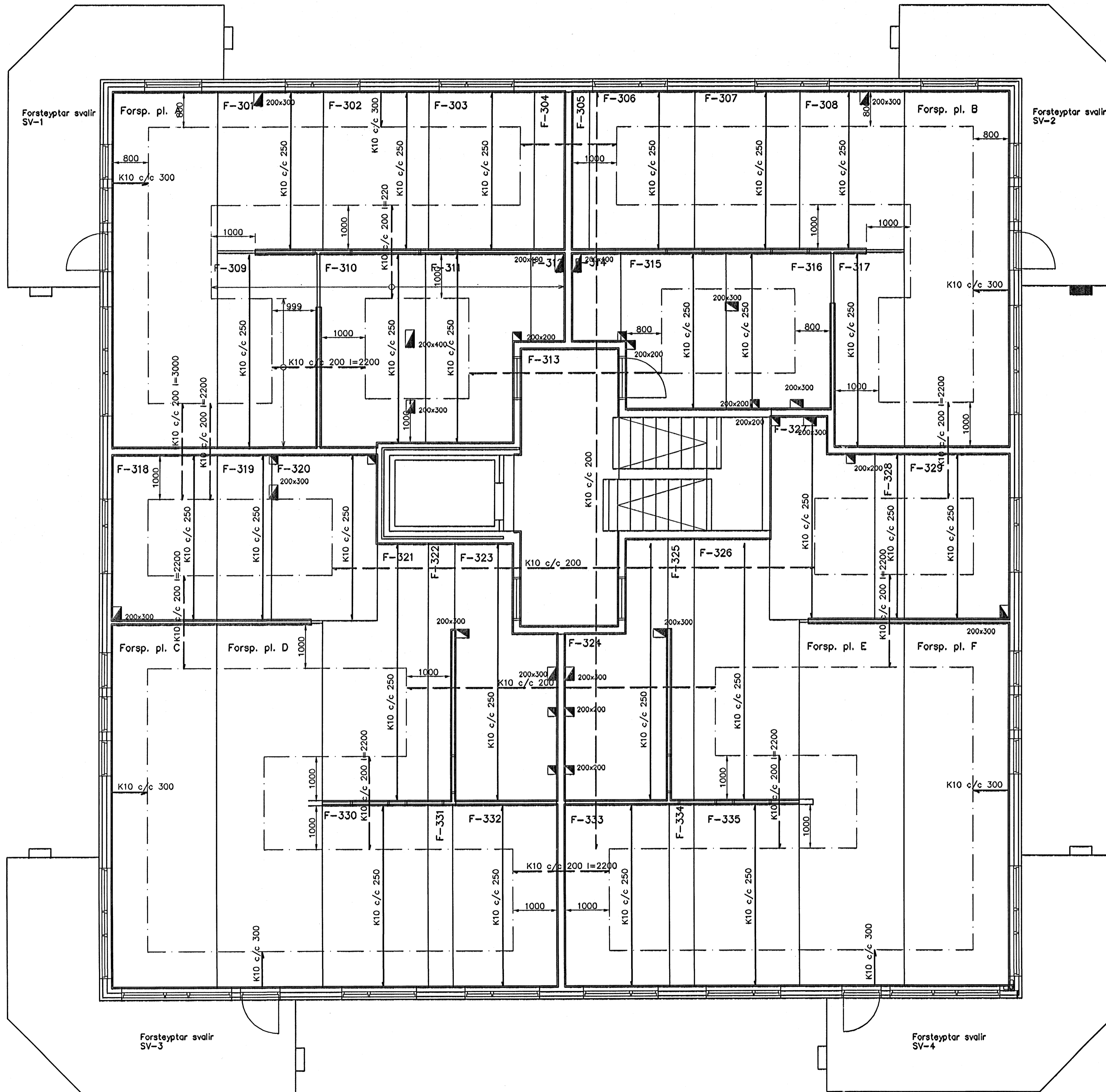
Plata yfir 2.hæð, Grunnmynd, 1:50
