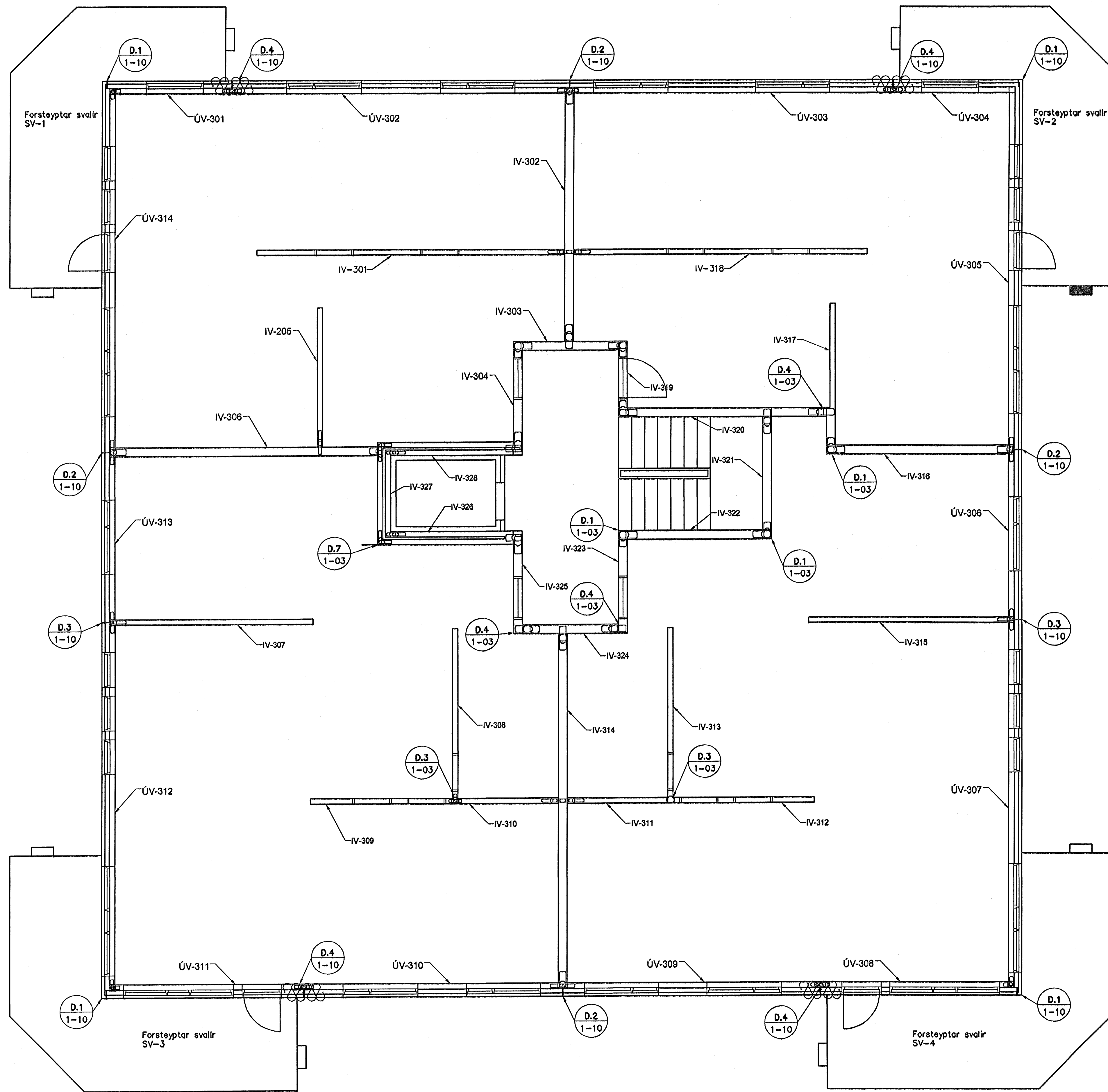
Veggir 2.hæð, Grunnmynd, 1:50
