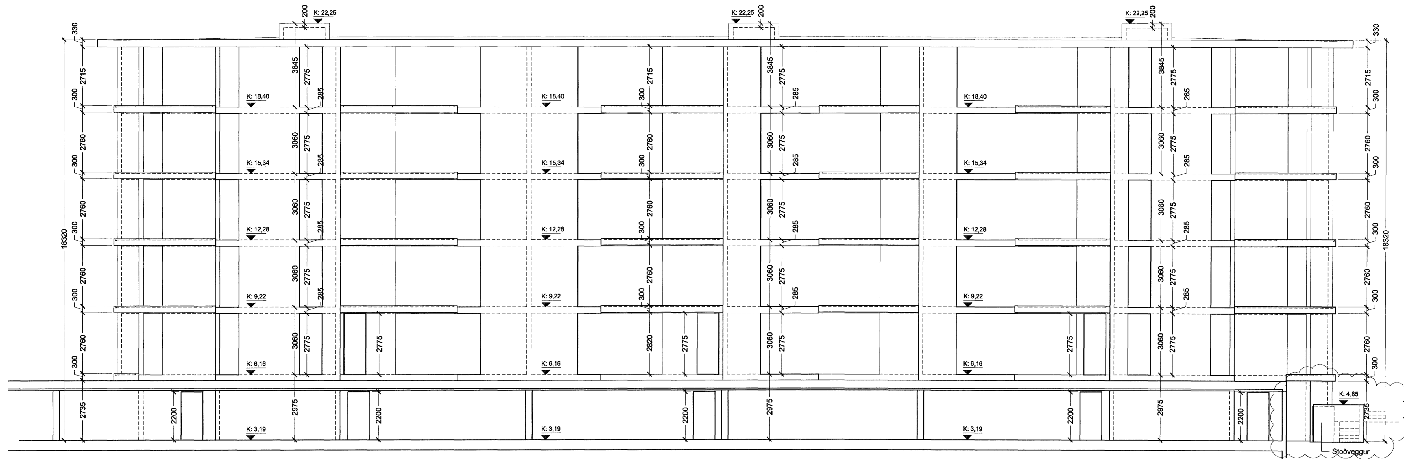
Vestur útlit í mkv. 1:100
