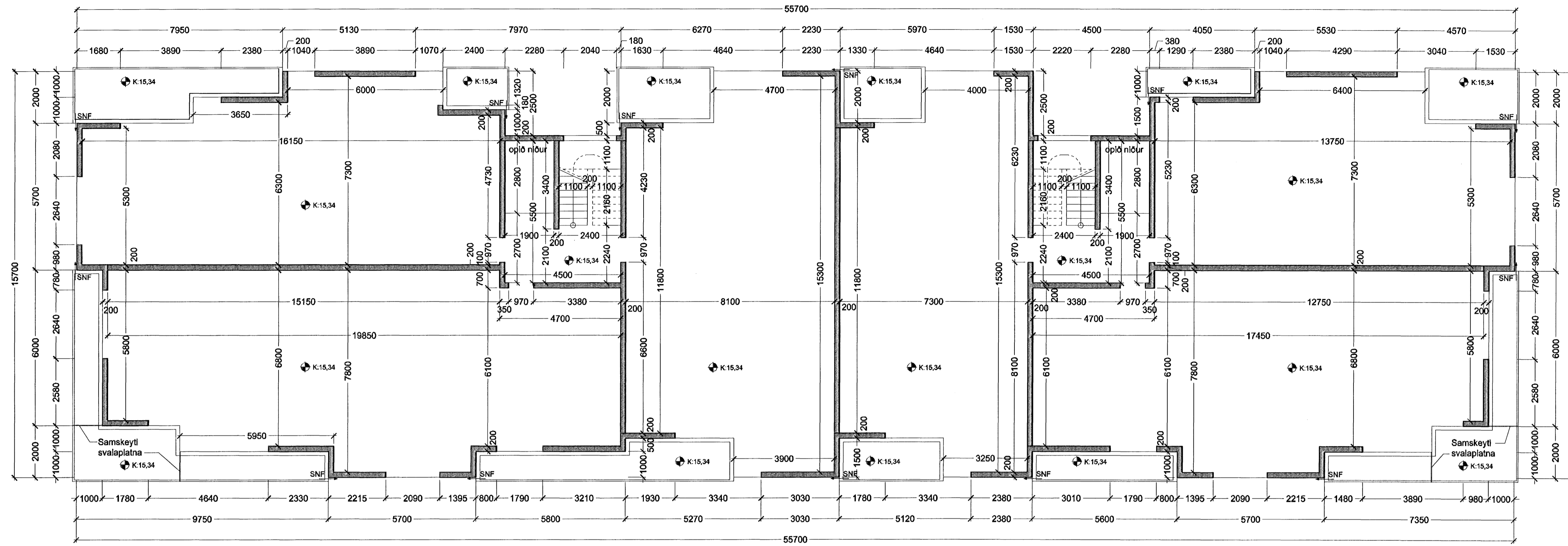
Grunnmynd 4. hæðar í mkv. 1:100
