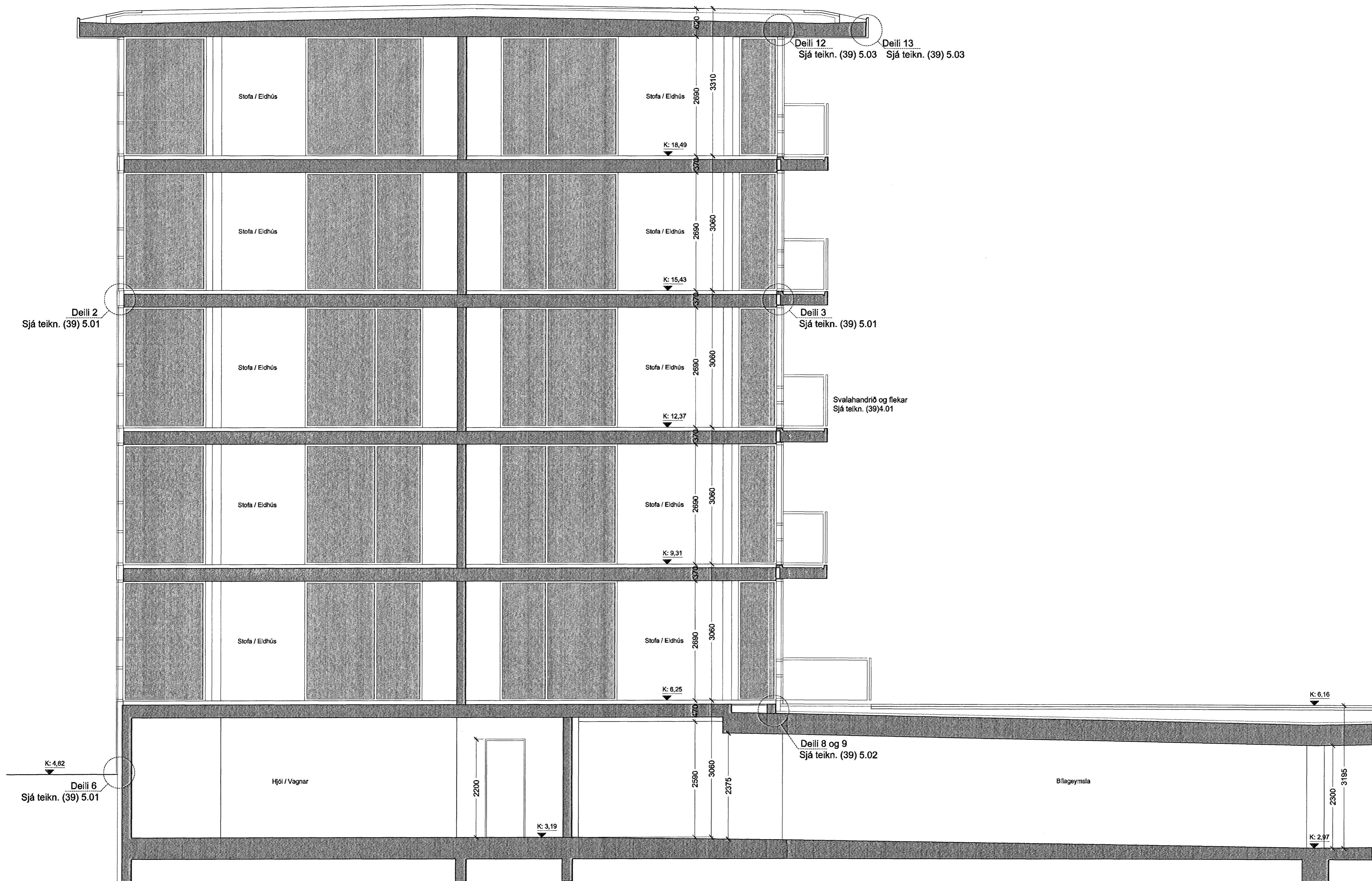
SNID B-B í mkv. 1:50
