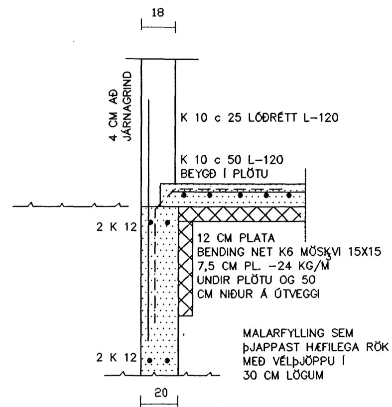
SNID - A 1:20 í ÚTVEGG-PLÖTU
