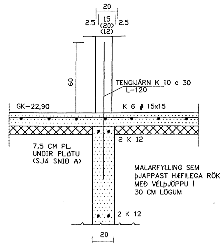
SNID - B 1:20 UNDIRSTÖÐUR INNVEGGJA
