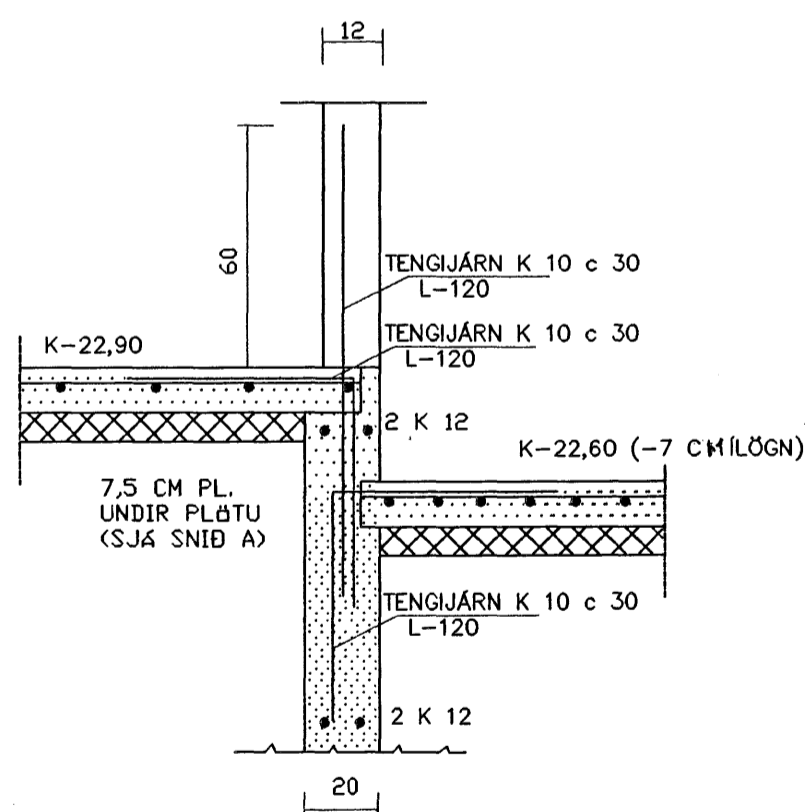
SNID - C 1:20 UNDIRSTÖÐUR INNVEGGJA
