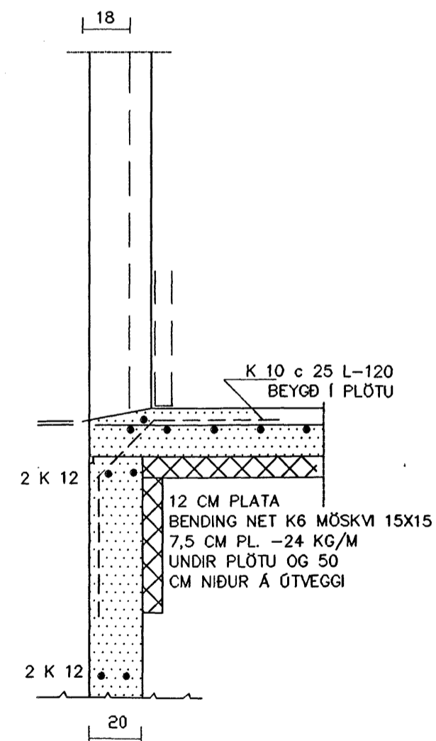
SNID - D 1:20 í ÚTVEGG VIÐ BÍLSKÜR
