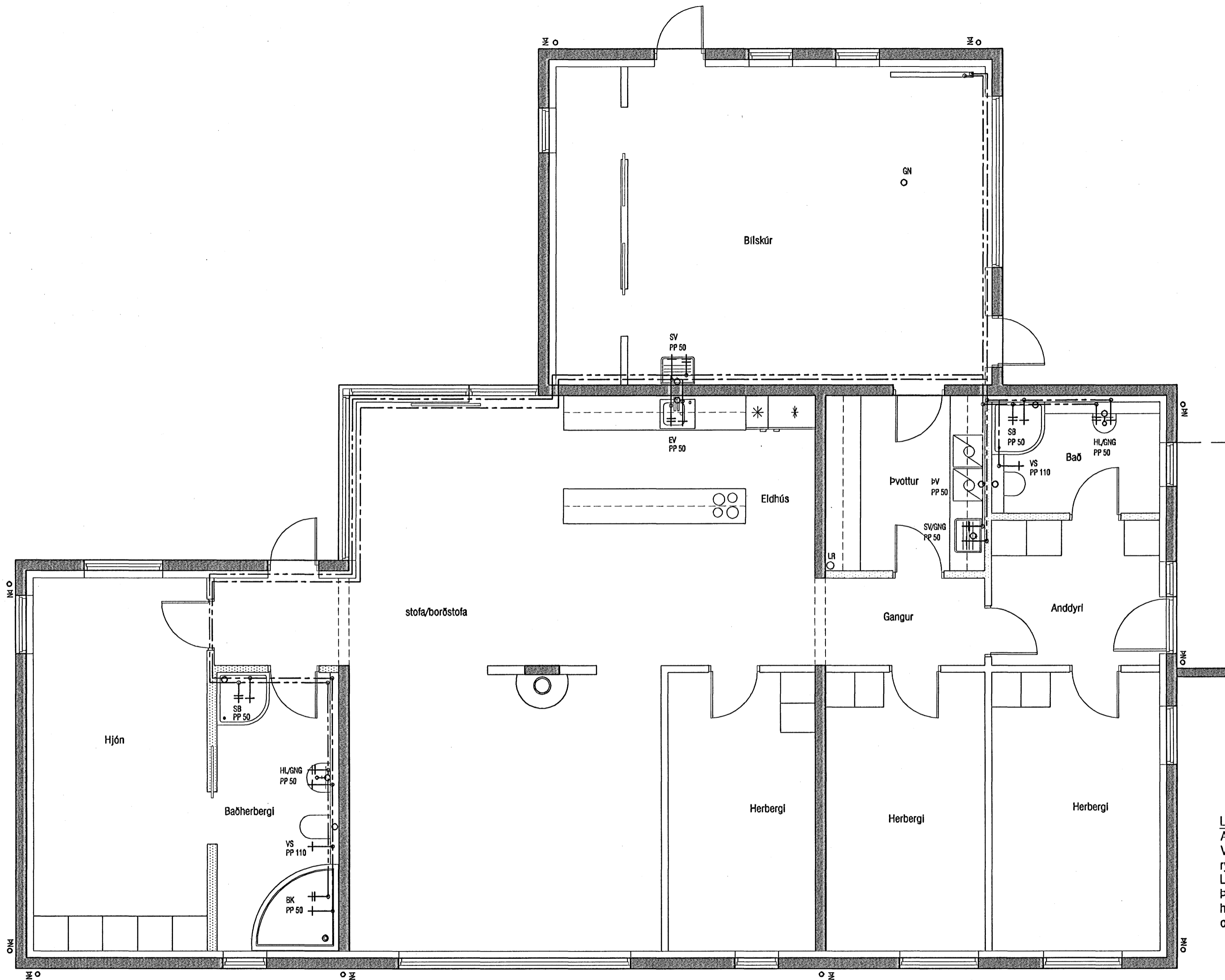
Grunnmynd
