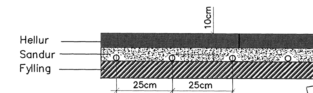
Snjóbræðslurör undir hellum Mkv. 1:10
