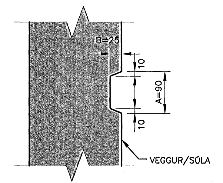
D08 DÆMIG. SKERLÁS, AxB
