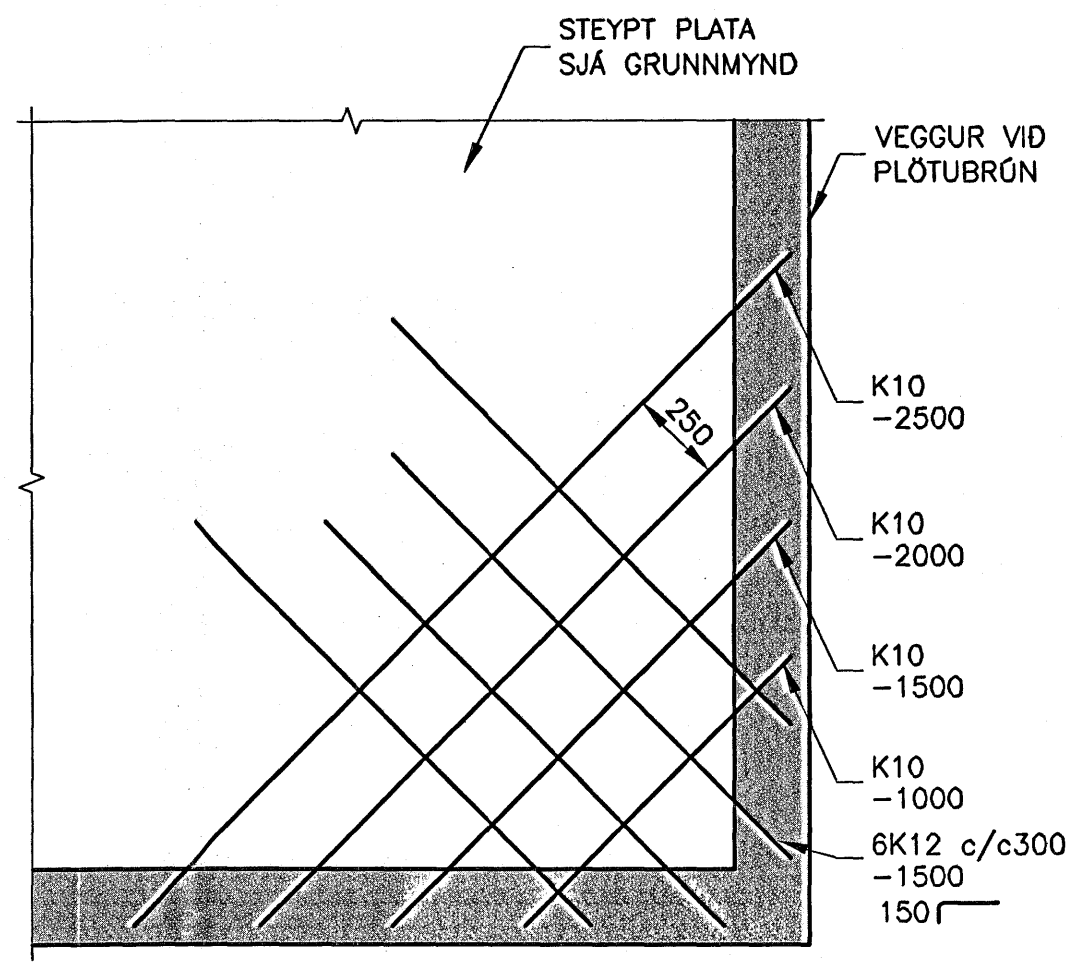
D07 JÁRNBENDING Í ÓUNDIRSTUDDRI PLÖTUBRÓN MKV. 1
