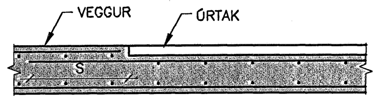
D09 JÁRNBENDING Í ÓRTAK Í VEGG MKV. 1
