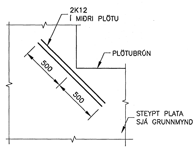
D06 JÁRNBENDING Í PLÖTUHORNÍ MKV. 1
