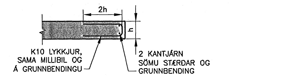
D07 JÁRNBENDING Í ÓUNDIRSTUDDRI PLÖTUBRÓN MKV. 1
