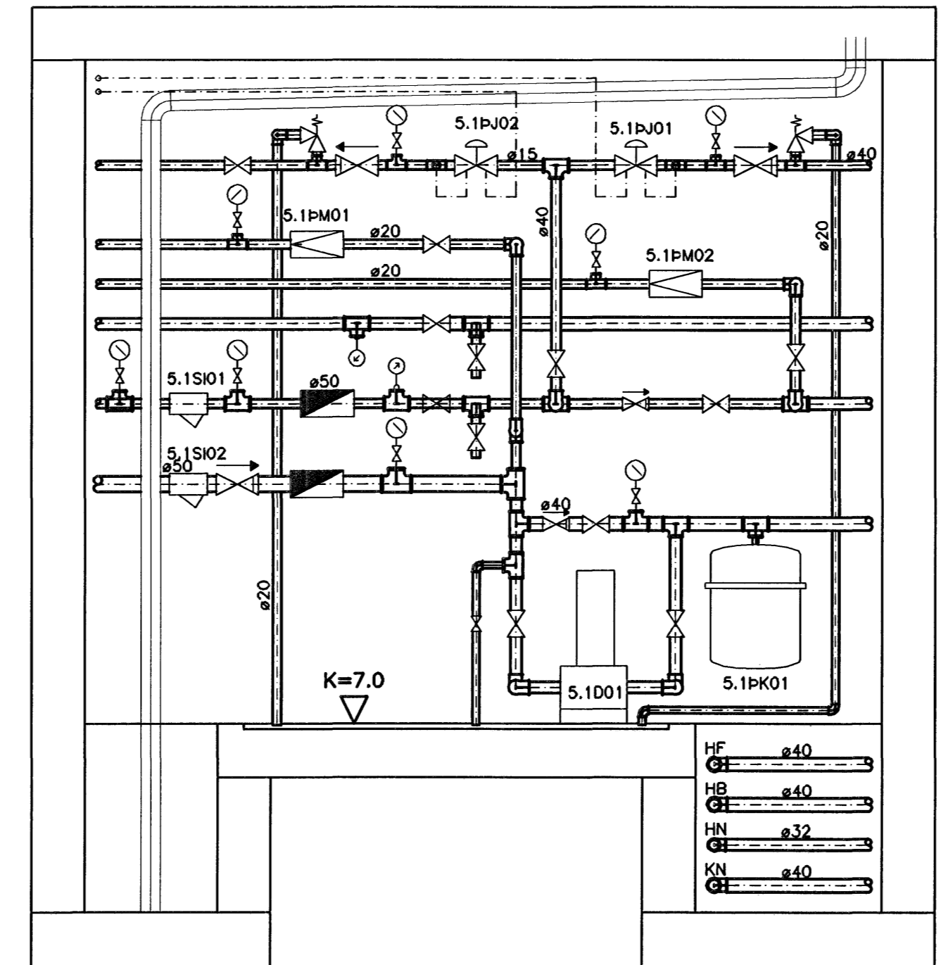
2 SNID-TENGIGRIND 10 14 26 M. 1:20
