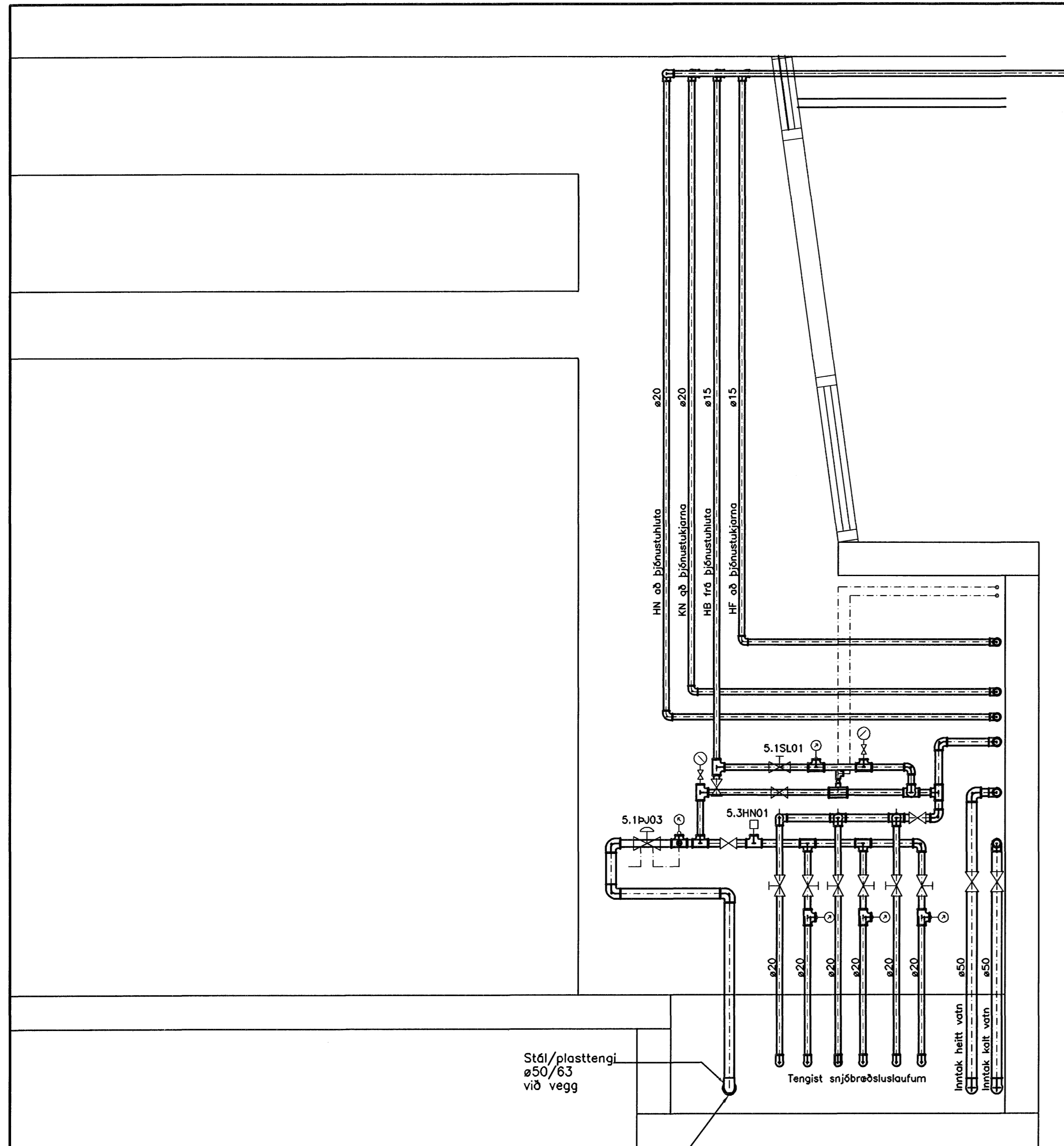
1 SNID-TENGIGRIND 14 26 M. 1:20
