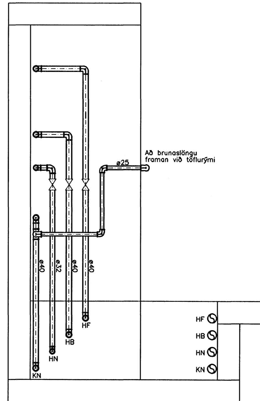
3 SNID-TENGIGRIND 14 26 M. 1:20
