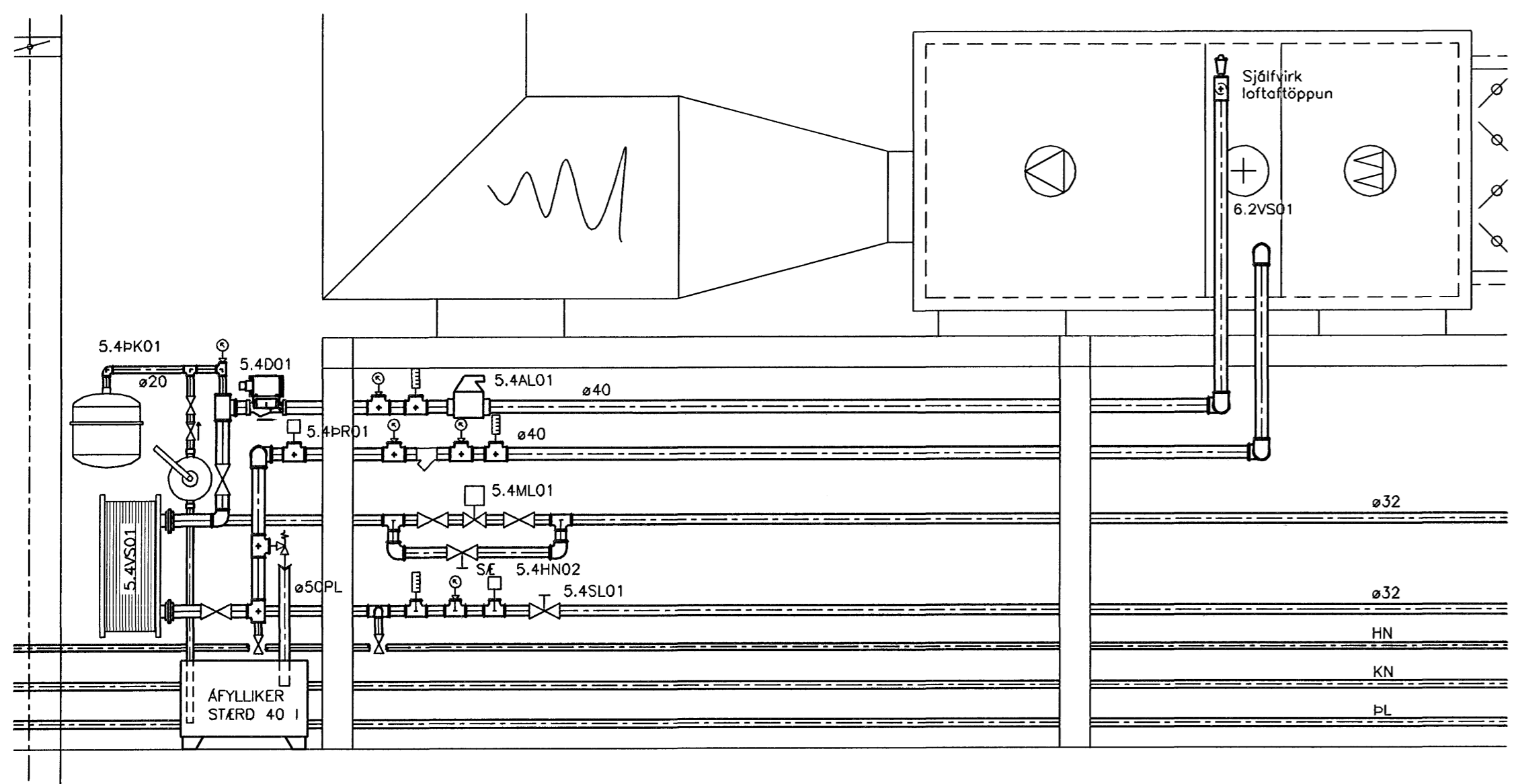
2 SNID-HITAKERFI LOFTRÆSINGAR 14 26 M. 1:20
