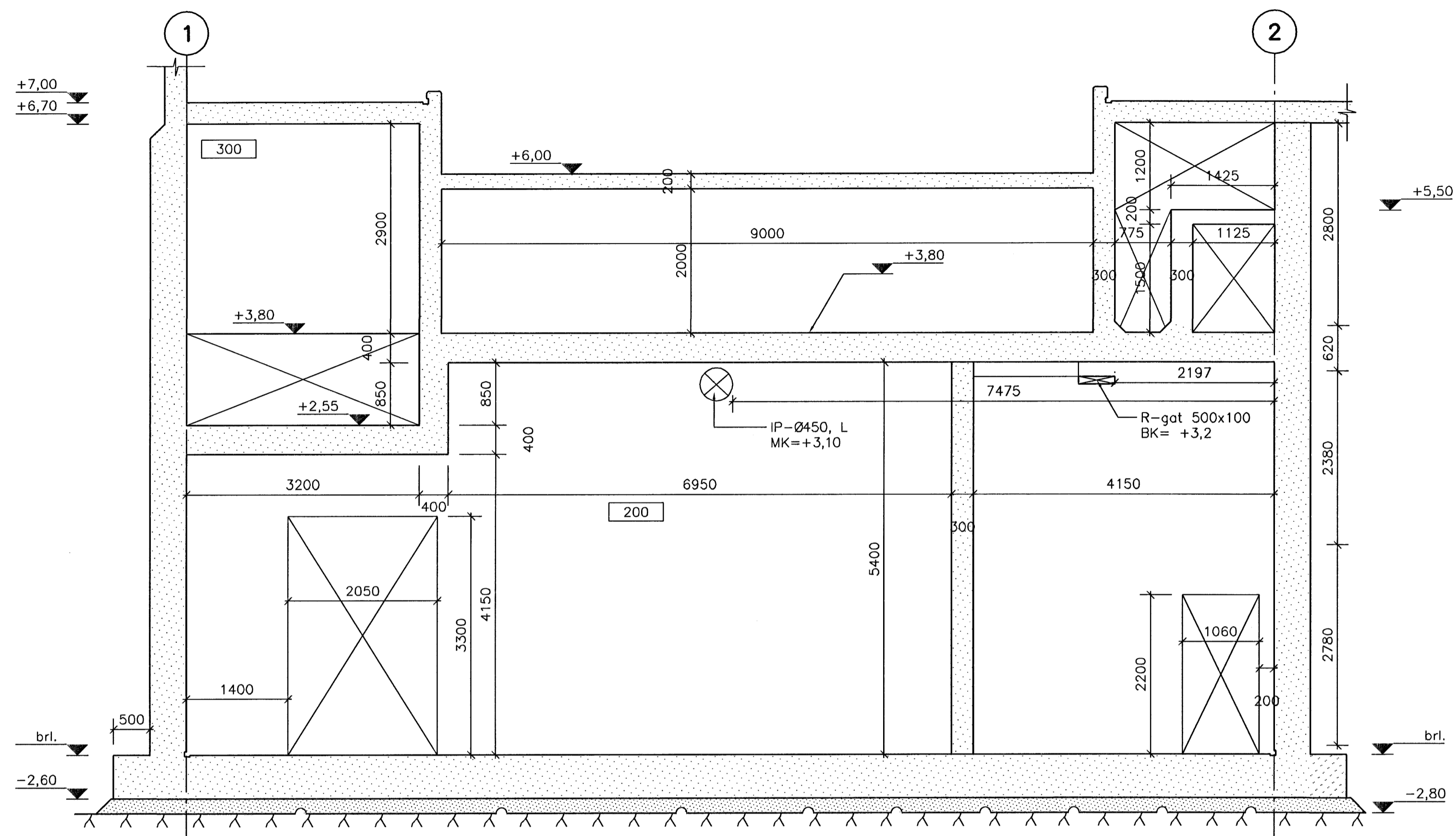
HLIDARMYND, VEGGUR Í LÍNU C -1,50 M. 1:50
