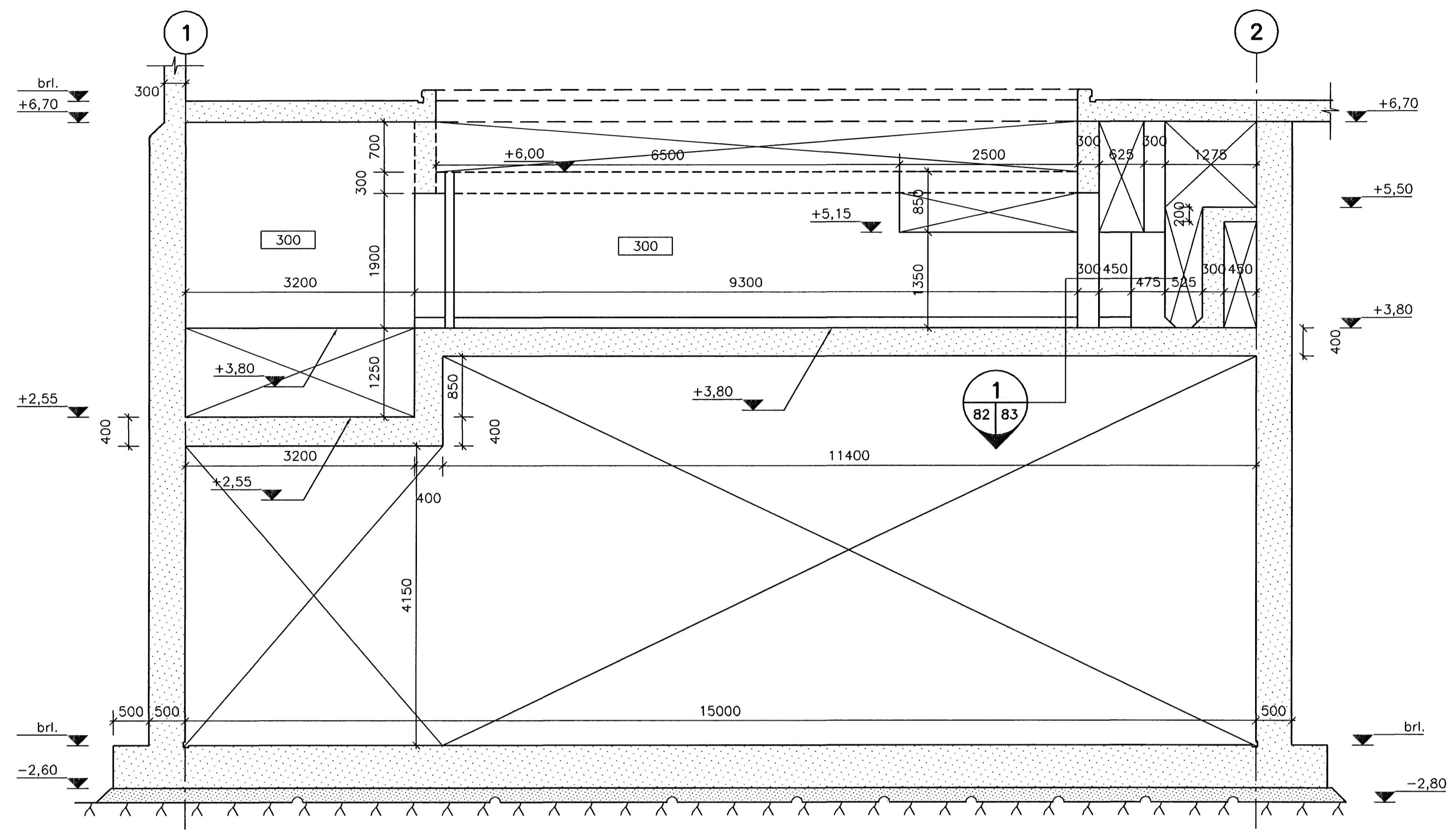
HLIDARMYND, VEGGUR Í LÍNU D +5,35 M. 1:50
