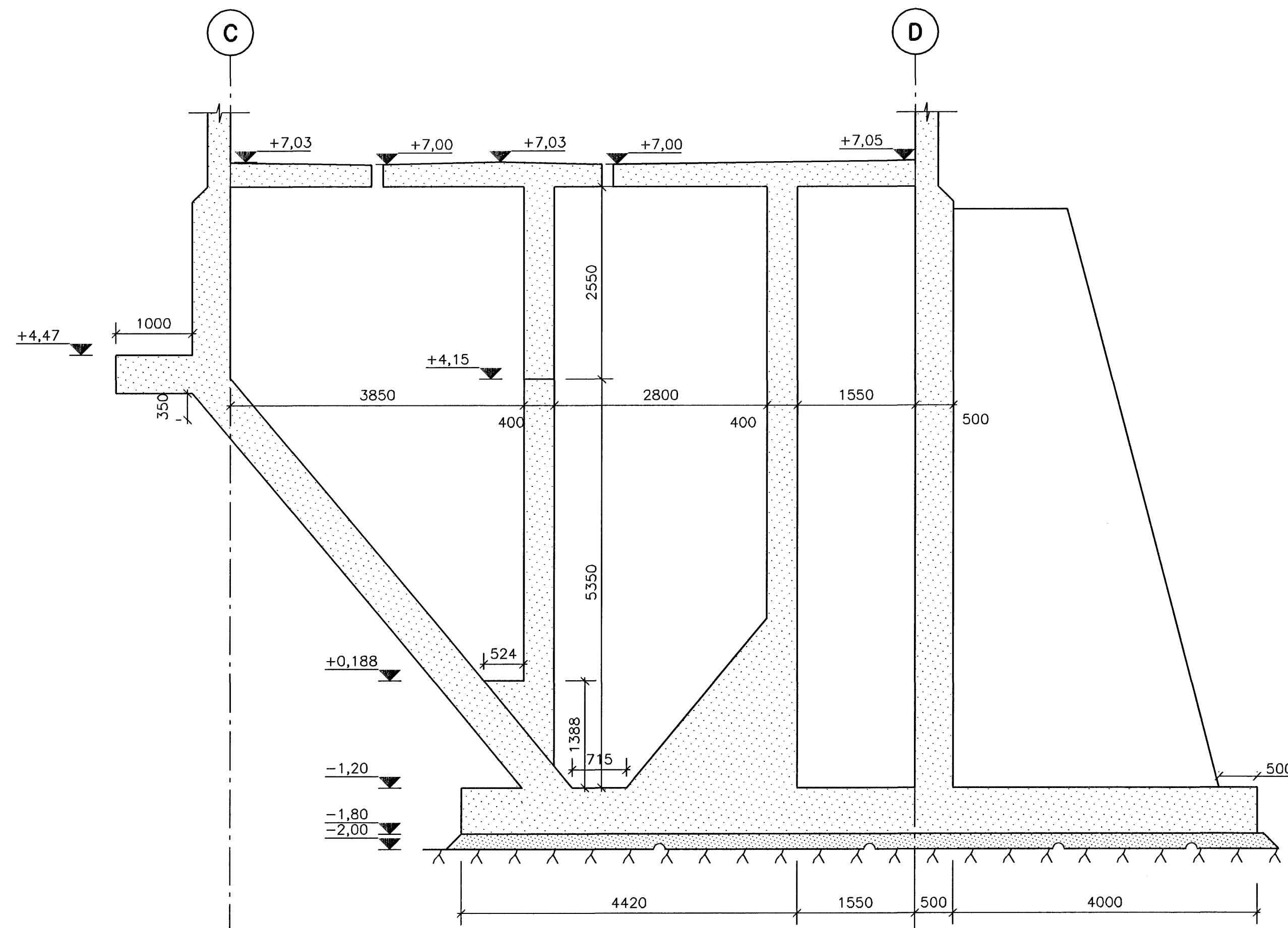
4 SNID 20 25 M. 1:50
