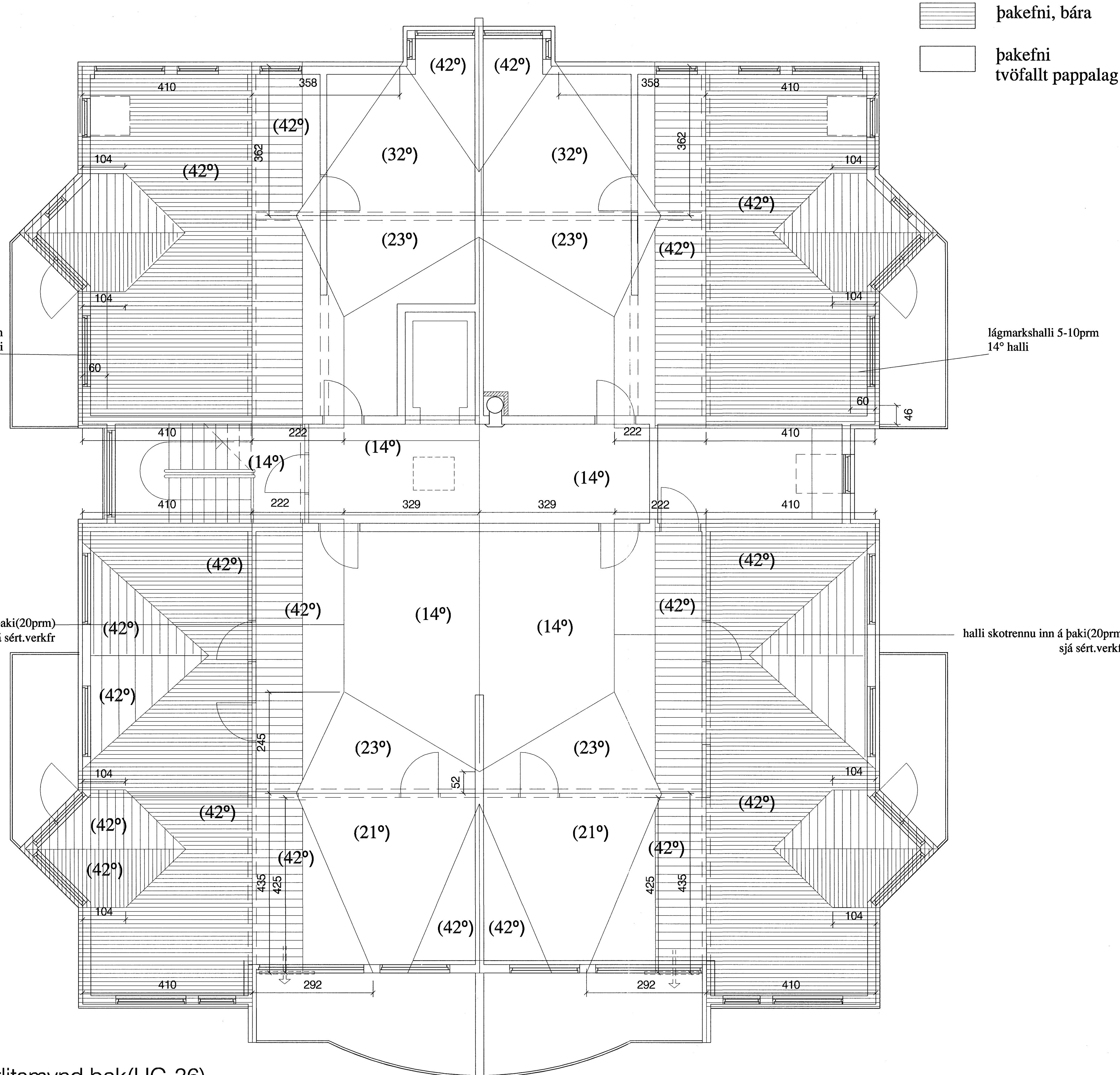
yfirlitsmynd þak(HG-36)
