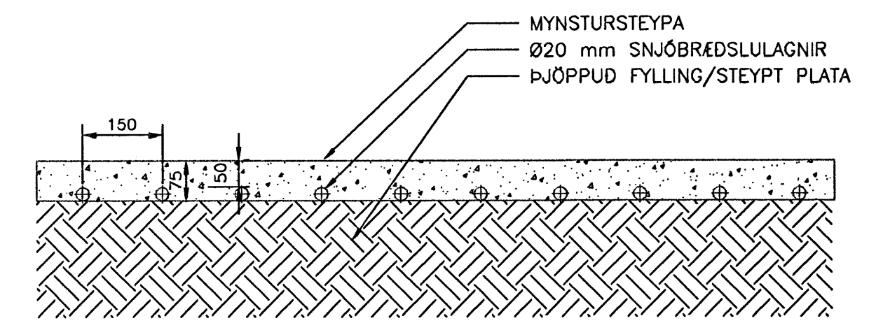
KENNISNIÐ SNJÓBR. Í MYNSTURSTEYPU 1:10
