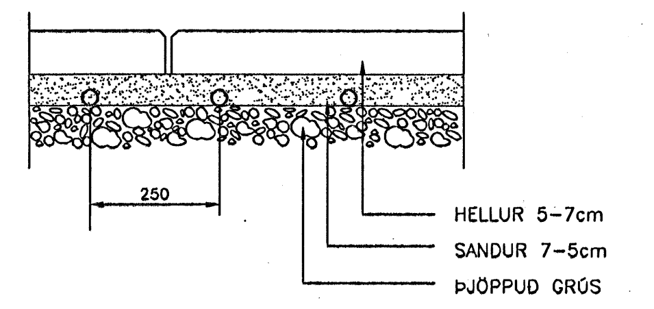
SNID Í HELLUR 1:10
