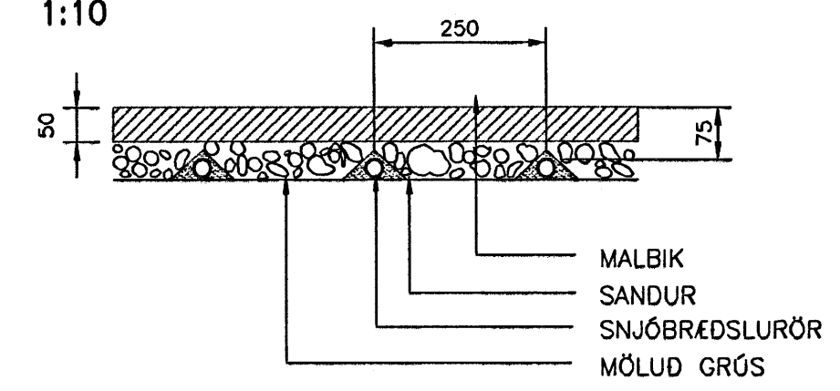
SNID Í MALBIK 1:10
