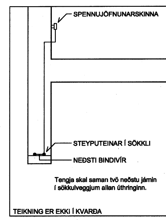
ÞVERSNIÐ Í SÖKKLI DÆMIGERÐUR FRÁGANGUR
