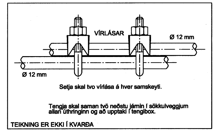
SAMTENGING STEYPUPEINA DÆMIGERÐUR FRÁGANGUR
