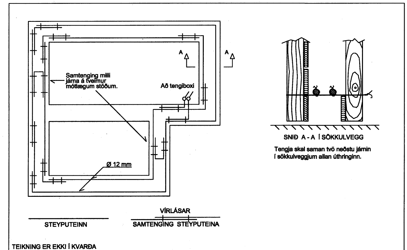
FYRIRMYND GRUNNMYND SÖKKULVEGGJA DÆMIGERÐUR FRÁGANGUR
