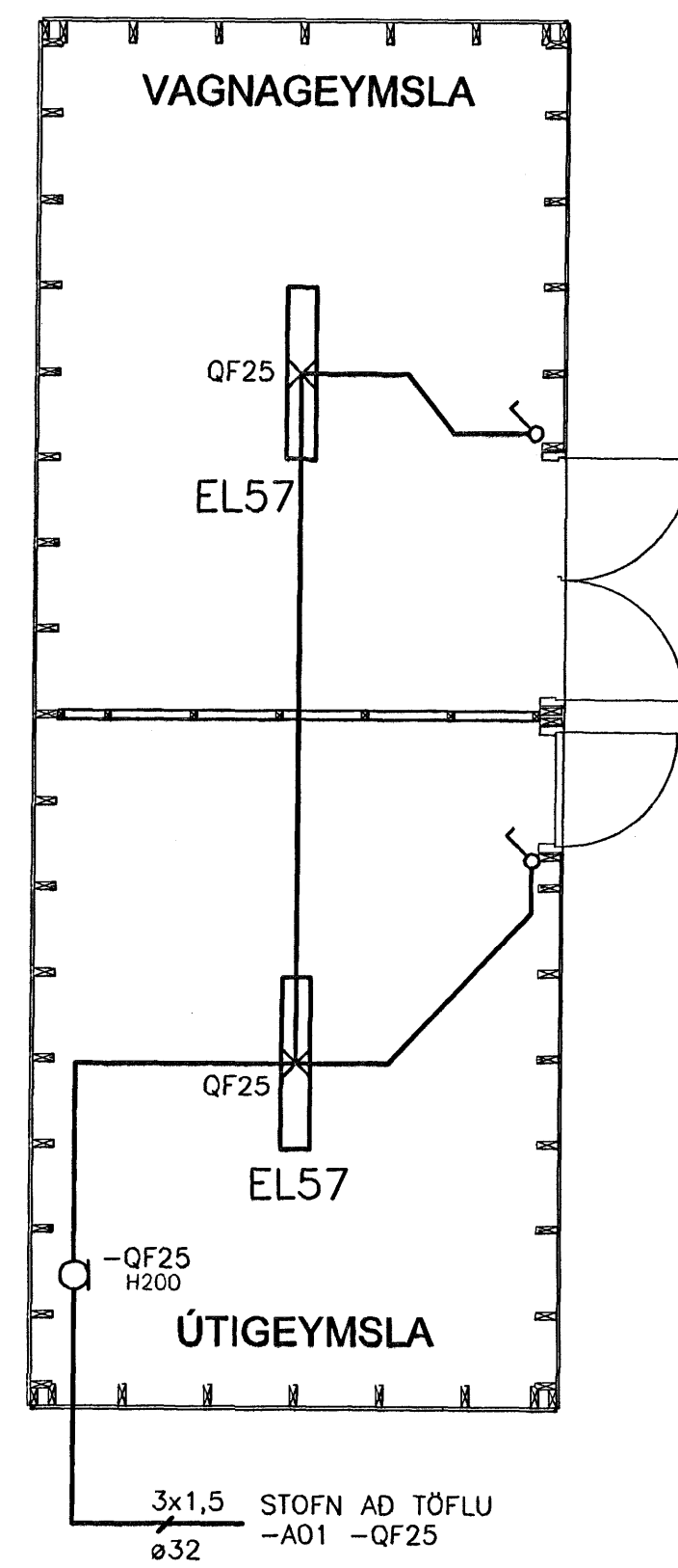
ÚTIGEYMSLA 1:50
