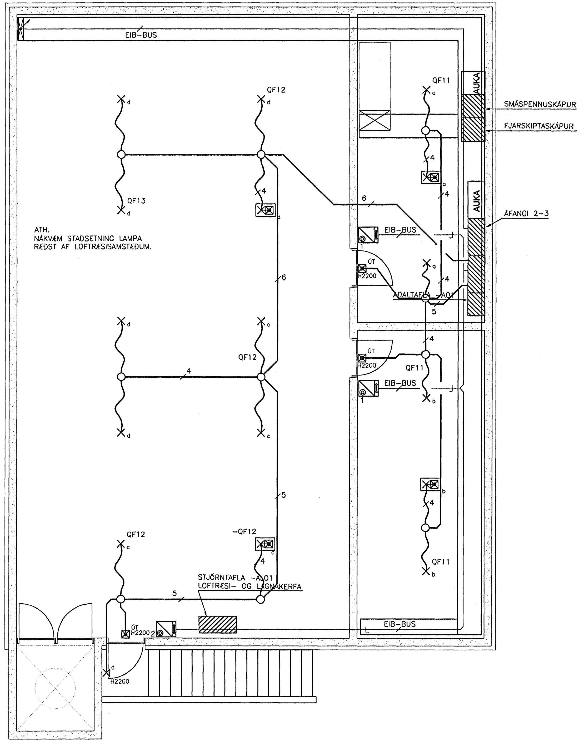
KJALLARI 1:50
