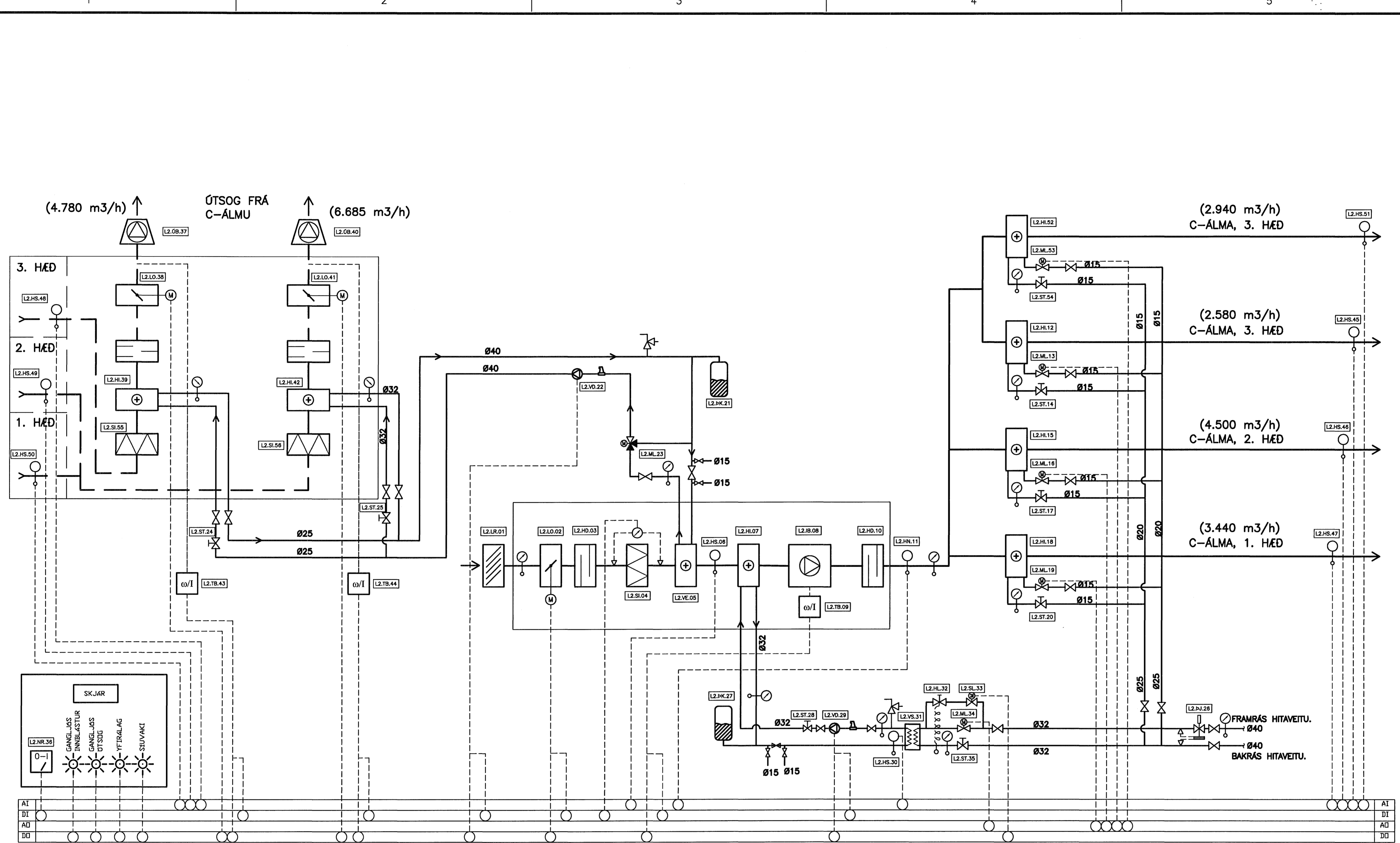
KERFISMYND FYRIR LOFTRÆSIKERFI L2
