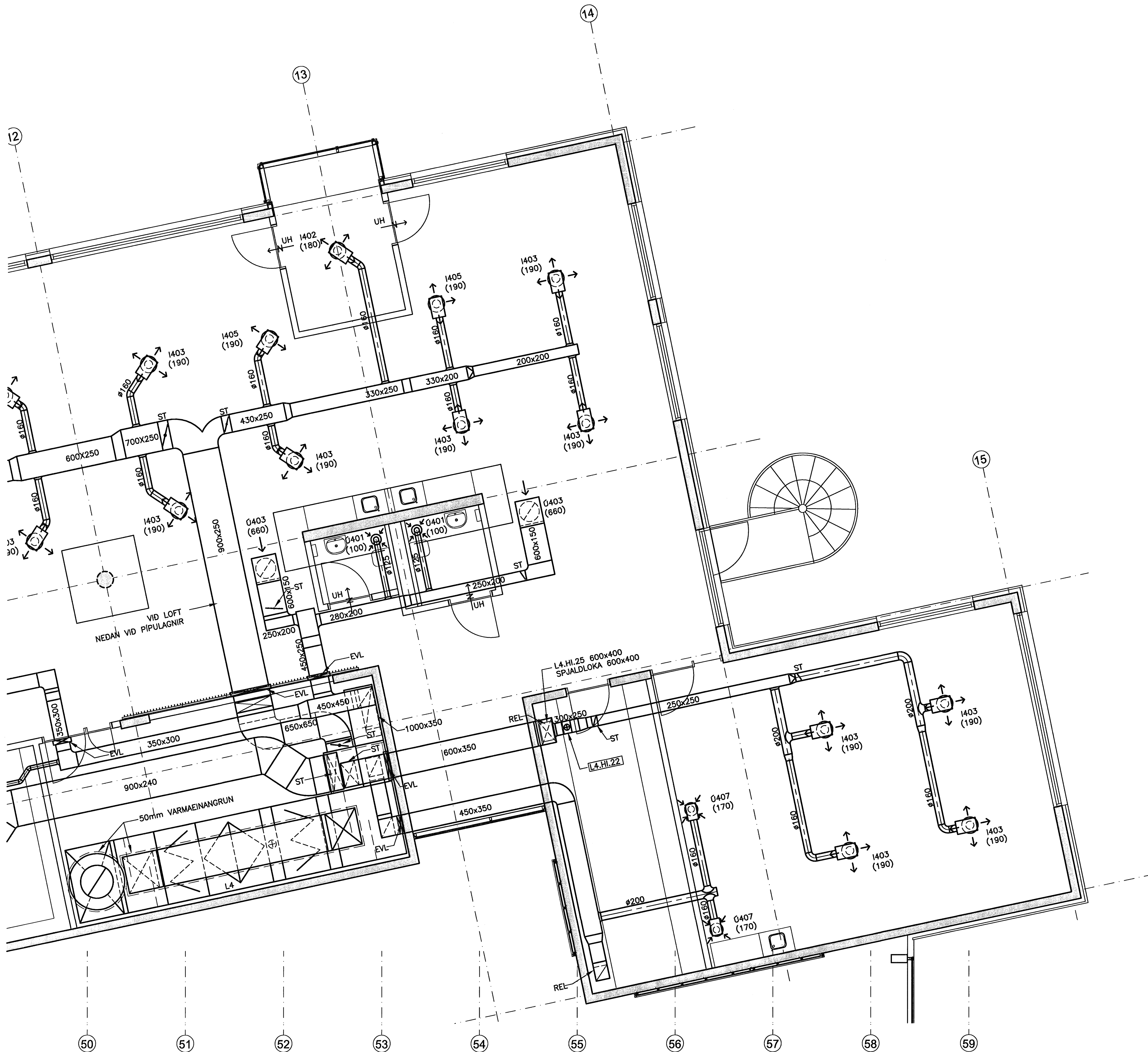
3. HÆÐ, GRUNNMÝND MKV. 1
