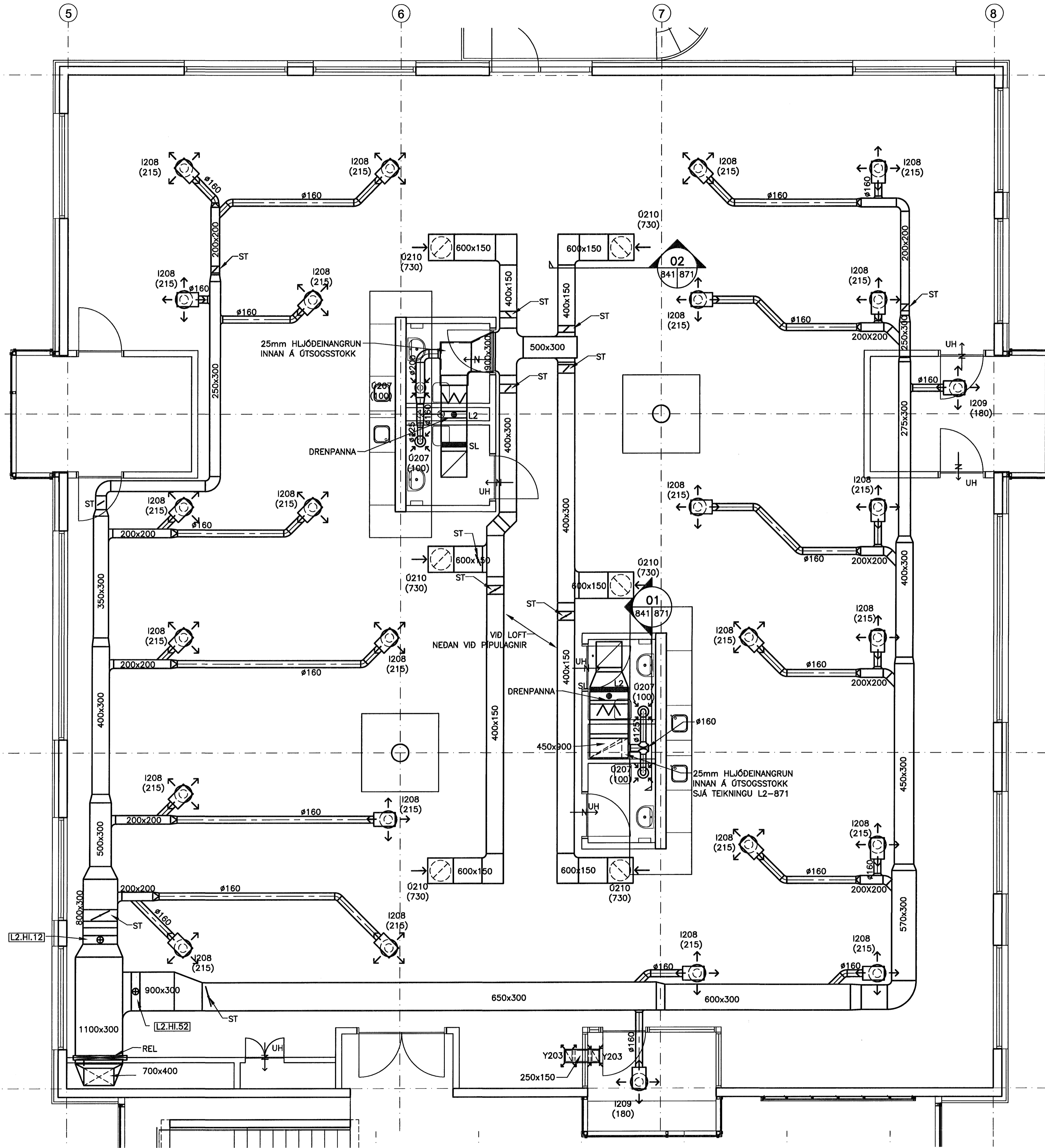
3. HÆÐ. GRUNNMYND MKV. 1
