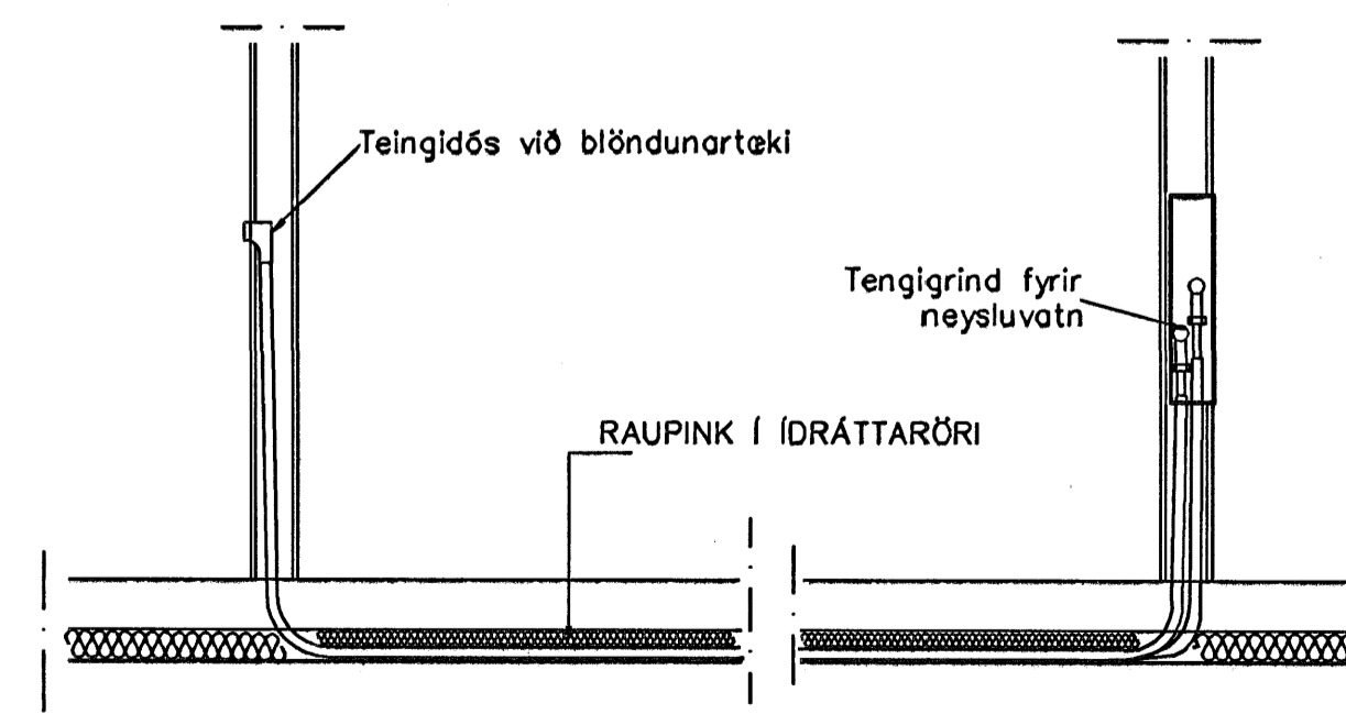
TENING NEYSLUVATNSLAGNA 1:20
