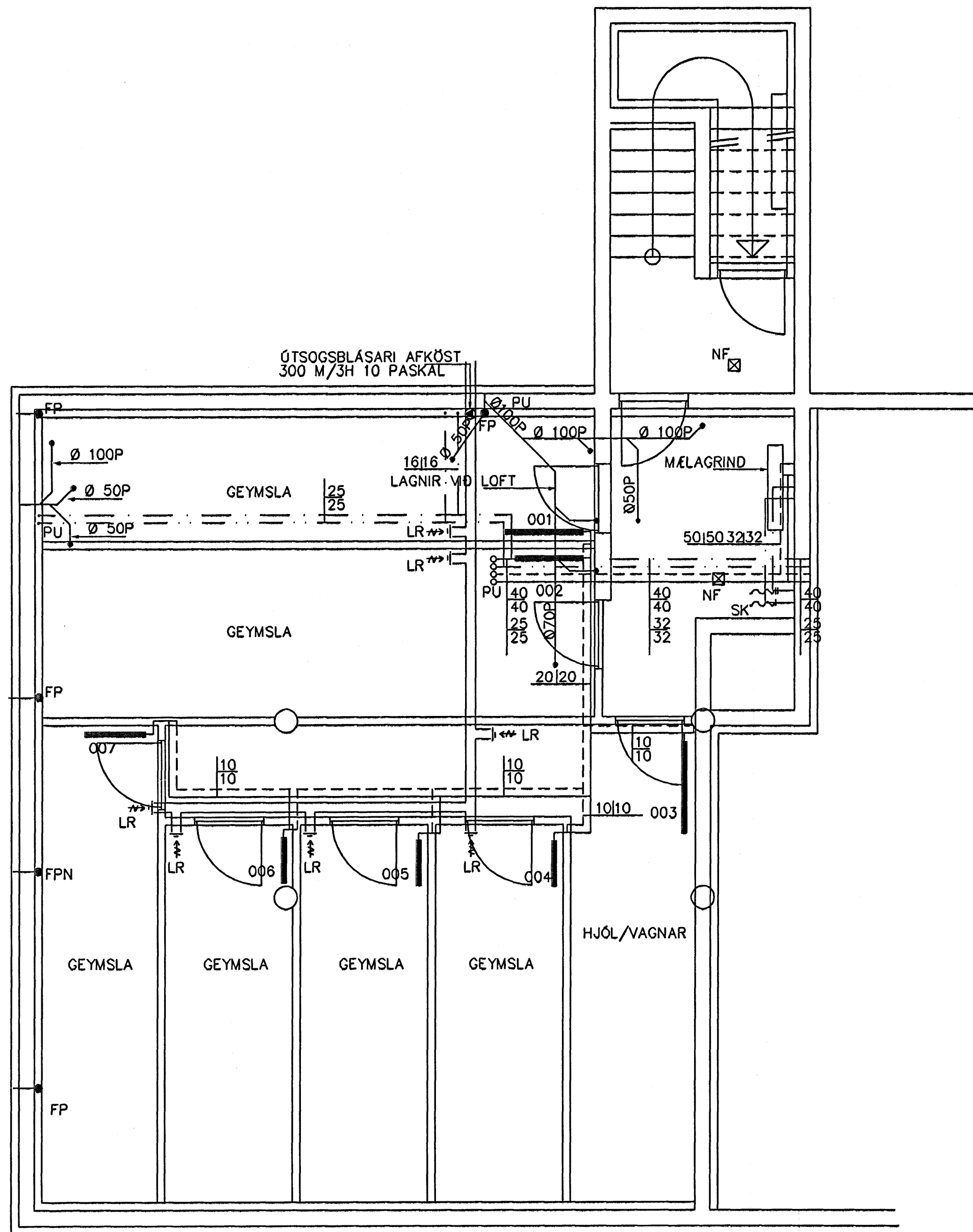
GRUNNMYND KJALLARA 1:50
