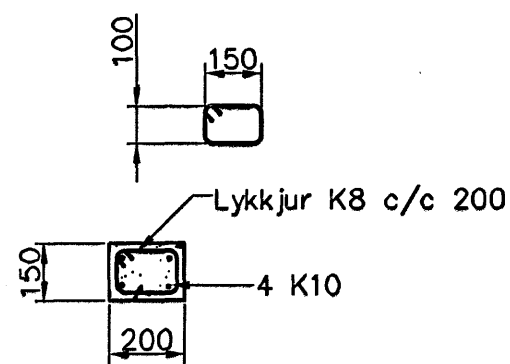
Súla S1.1 1:20 1-02
