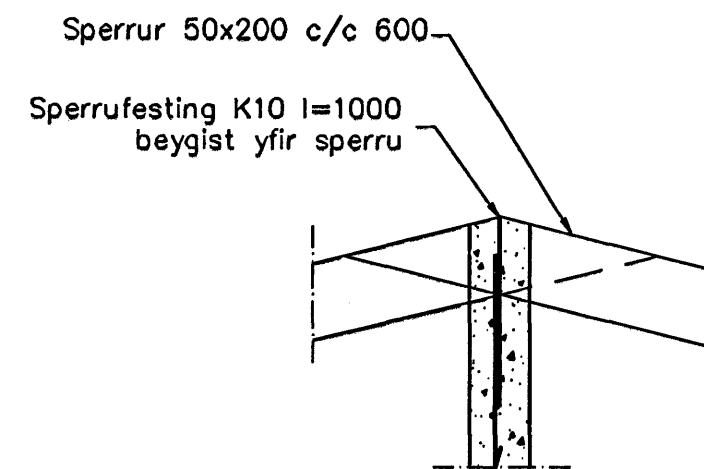
Snið 2 1:20 1-01
