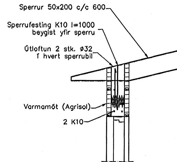
Snið 1 1:20 1-01
