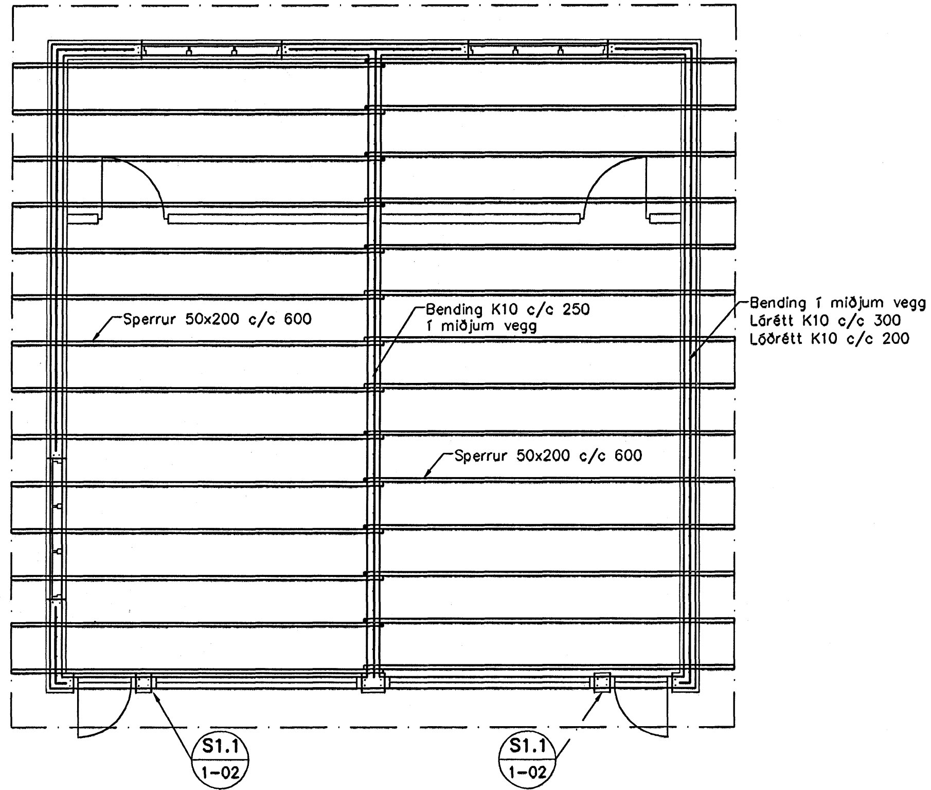
Veggir, þak, Grunnmynd, 1:50
