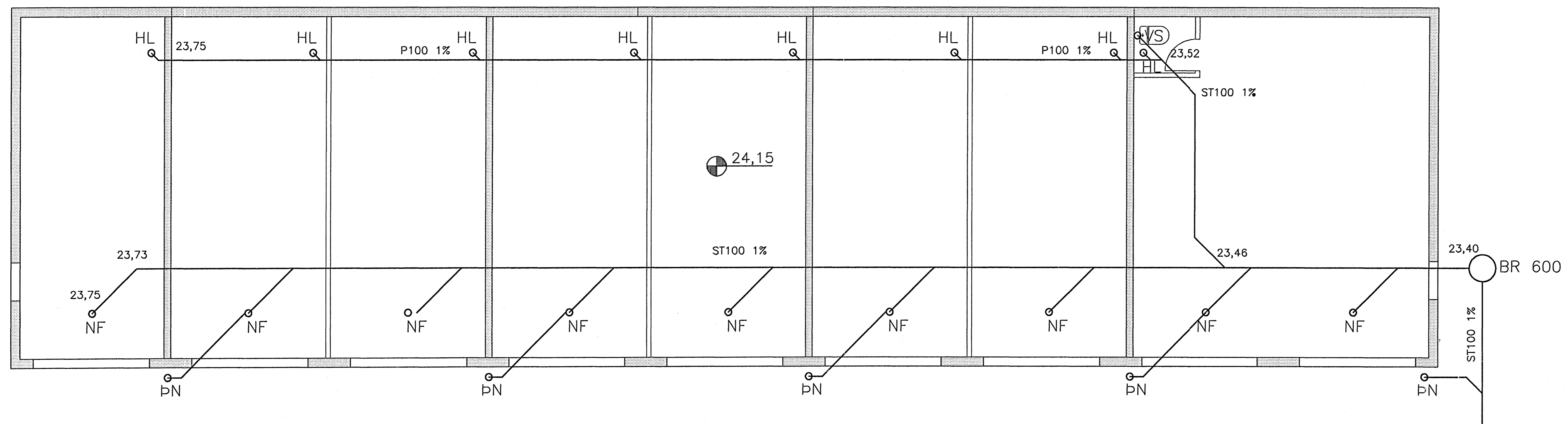
GRUNNMYND 1:50
