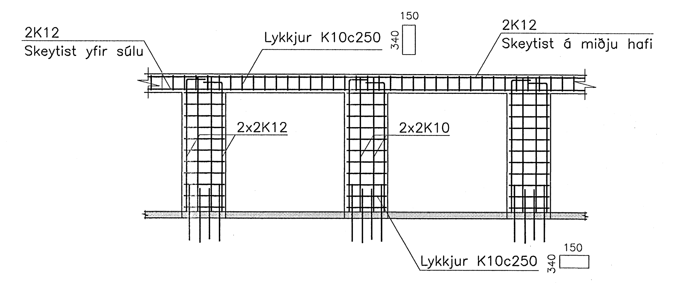
ASÝND E 1.50
