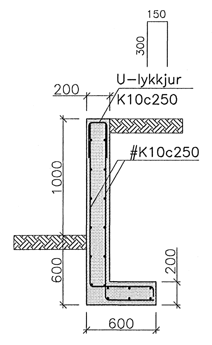
SNID D 1:20
