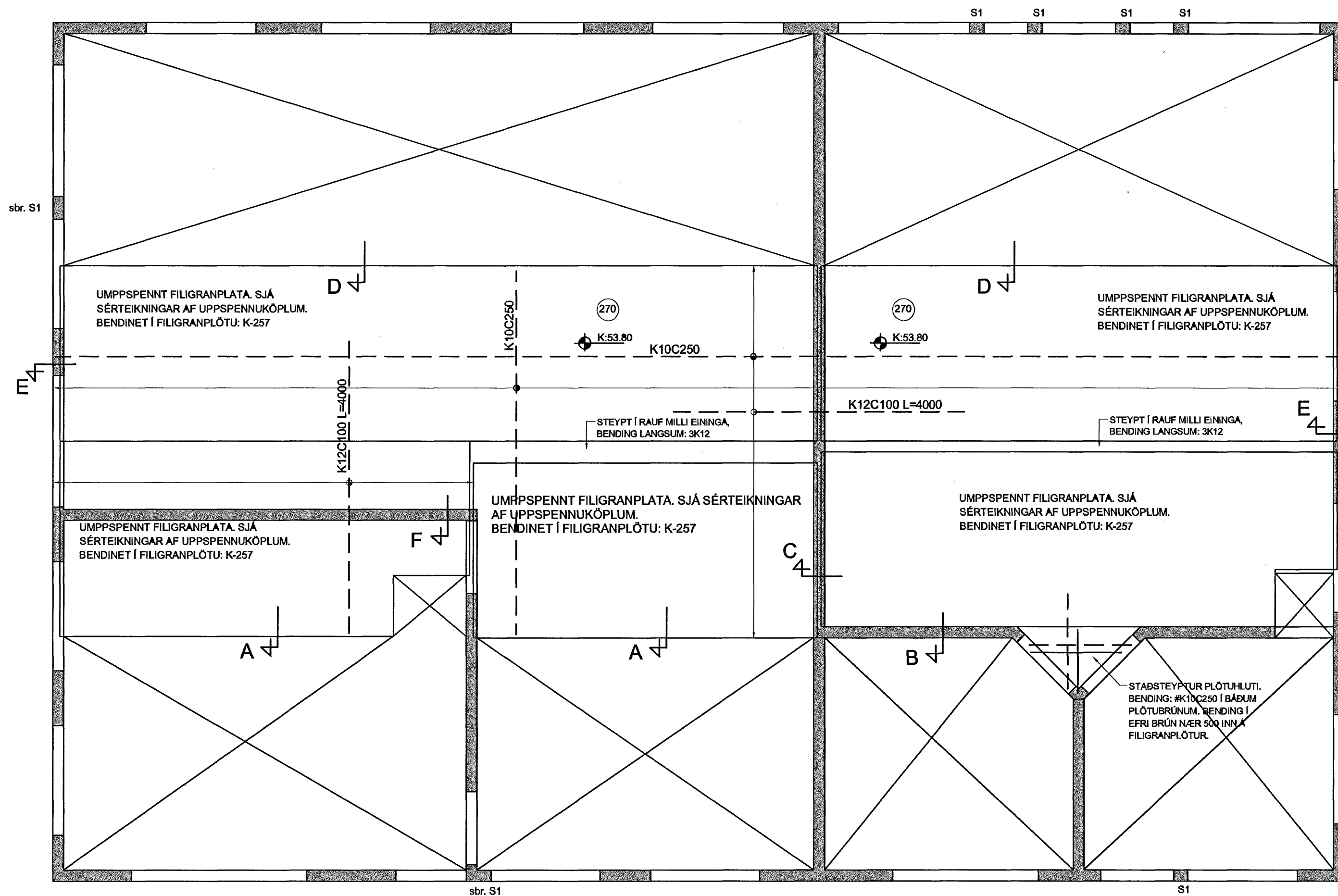
GRUNNMYND PLÖTU YFIR 1. HÆÐ, 1:50
