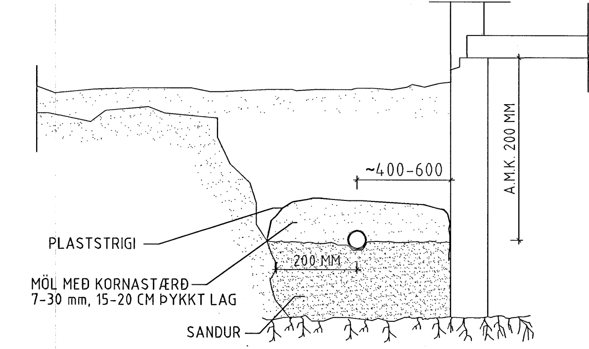
DÆMIGERT SNIÐ Í FRÁGANG PERRILAGNA, 1:20
