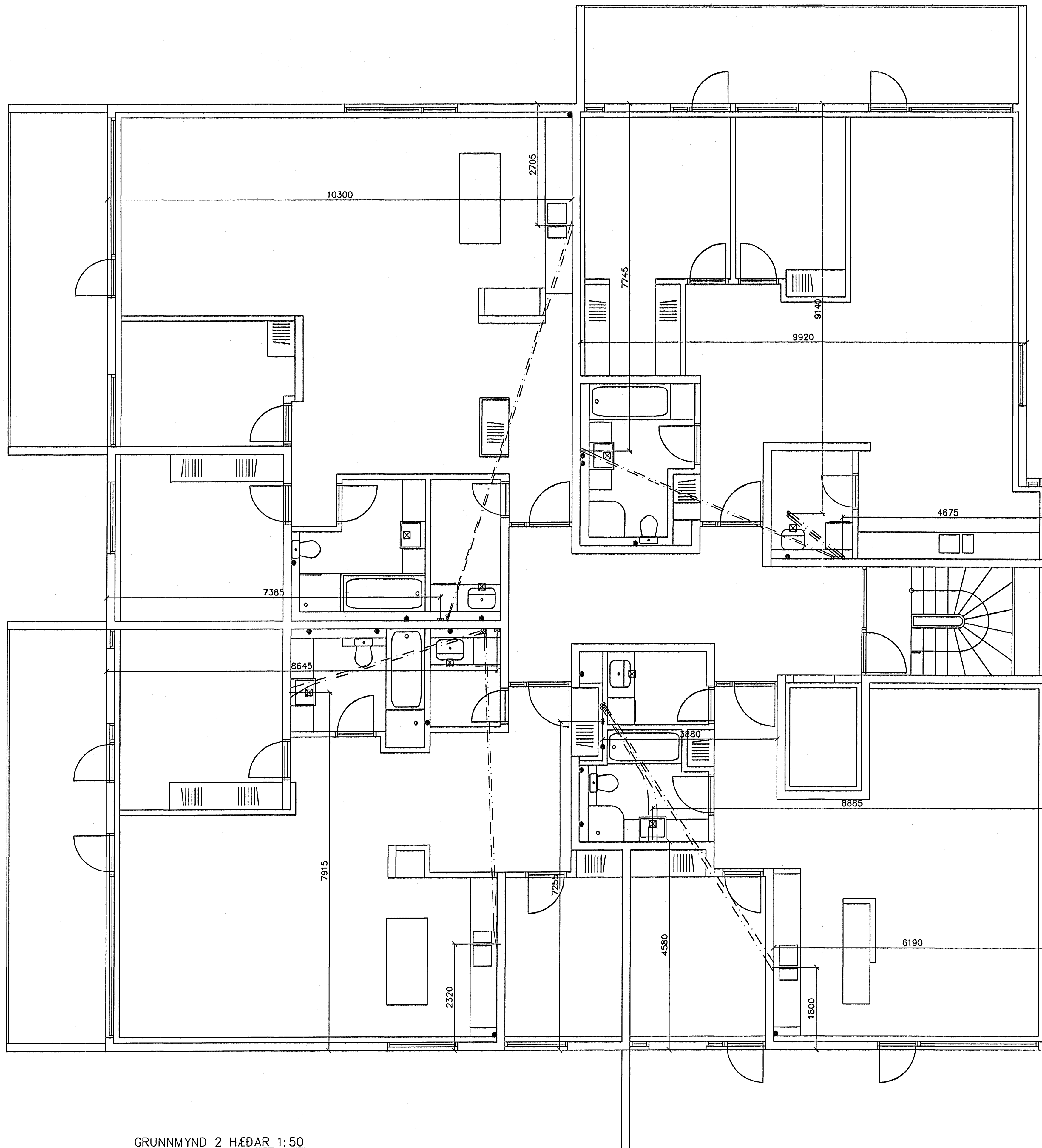
GRUNNMYND 2 HÆÐAR 1:50
