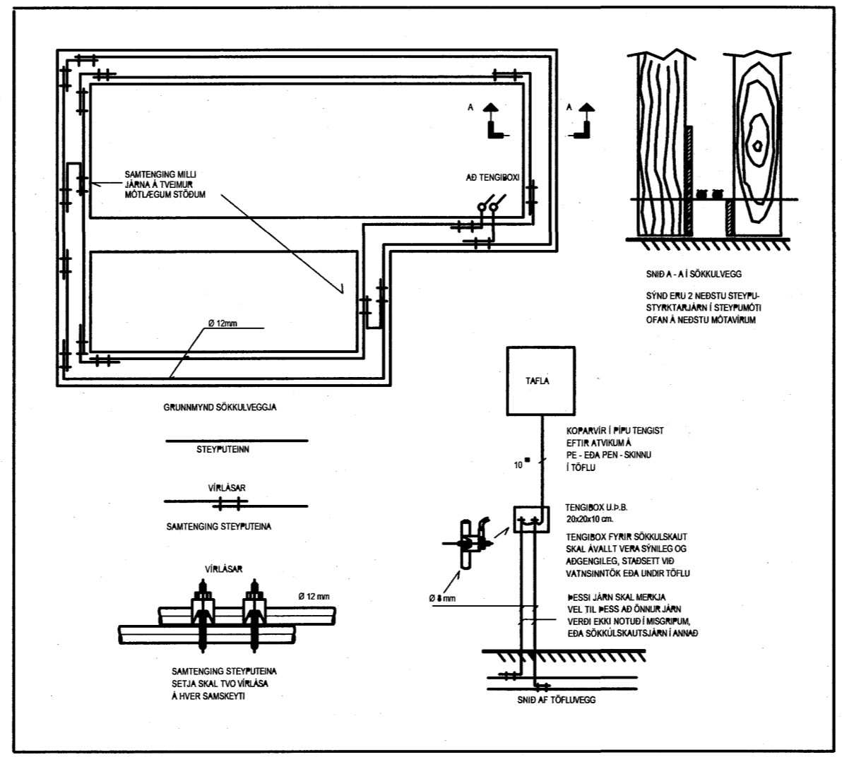
Skýringarmynd sökkulskaut
