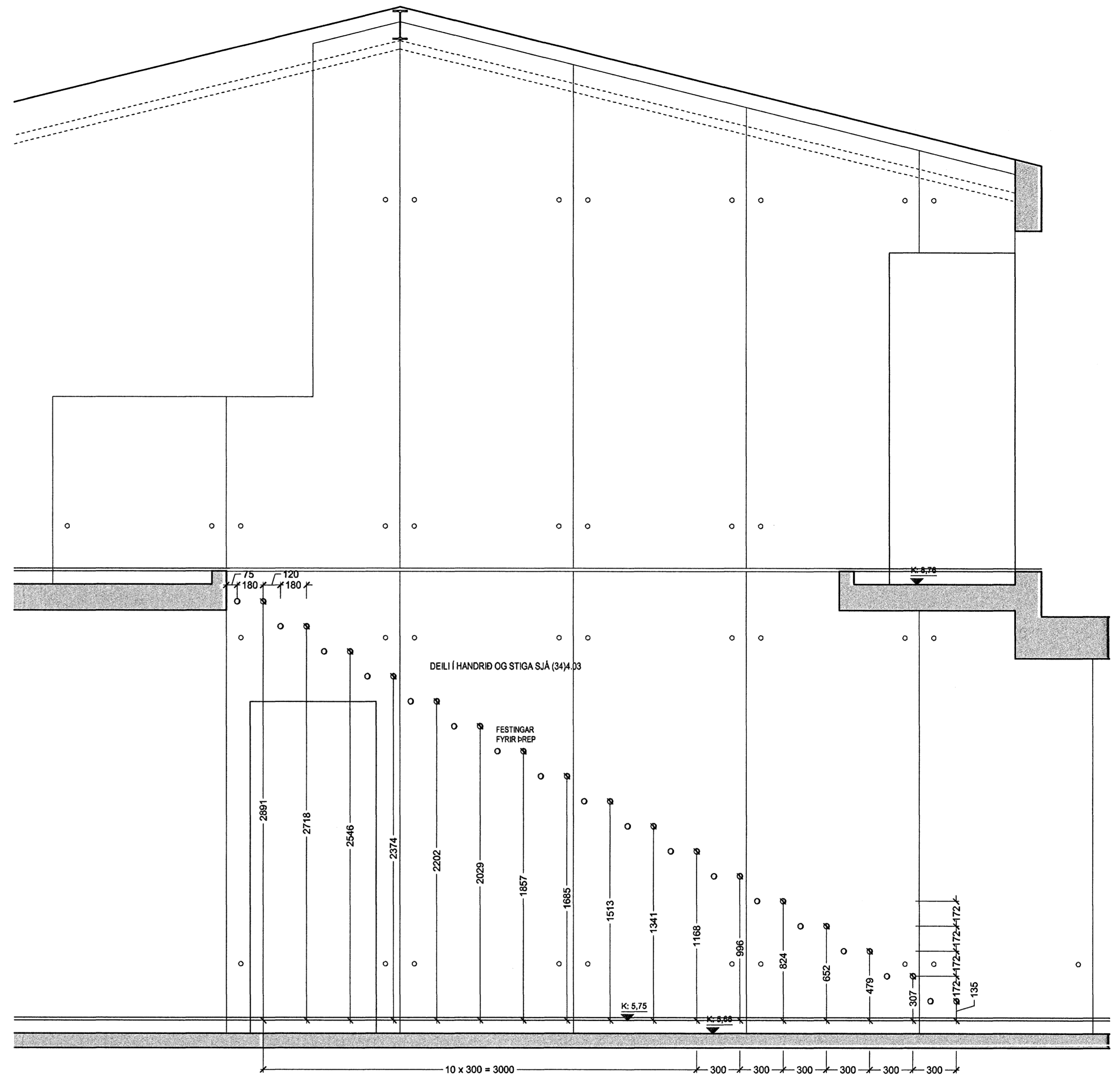
ÁSYND FESTINGAR STIGI MKV 1:20
