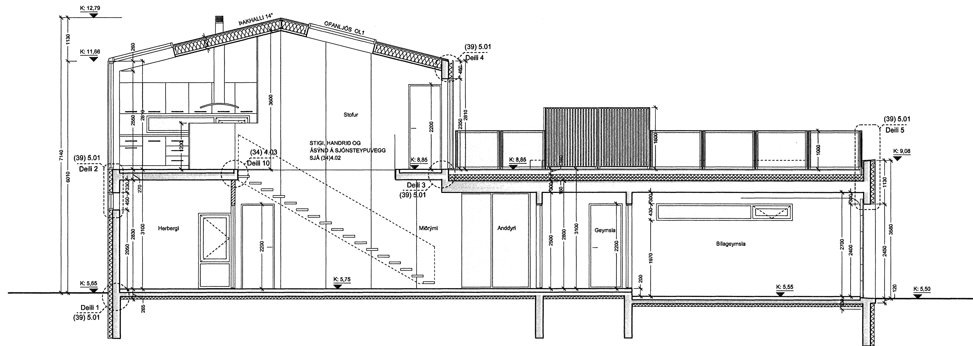
SNID A-A MKV 1:50
