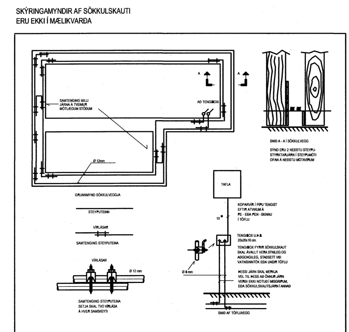
Skýringarmynd sökkulskaut
