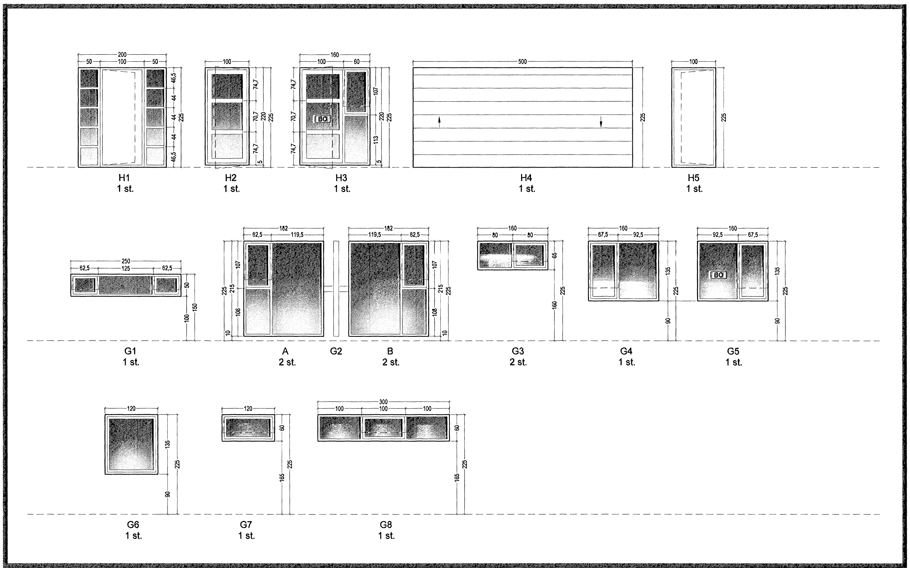
Gluggateikning 1:50
