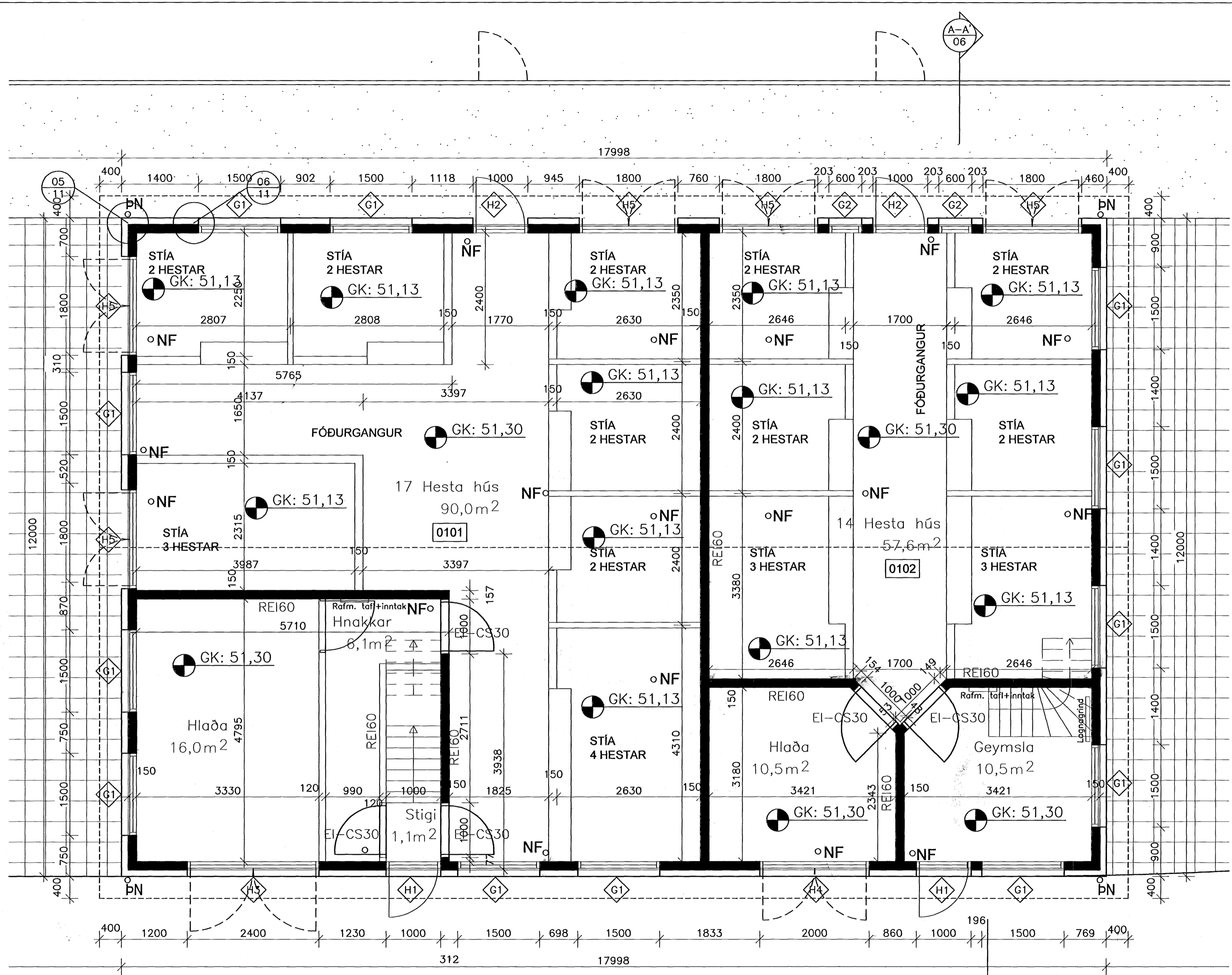
GRUNNMYND 1. HÆÐAR 1:50
