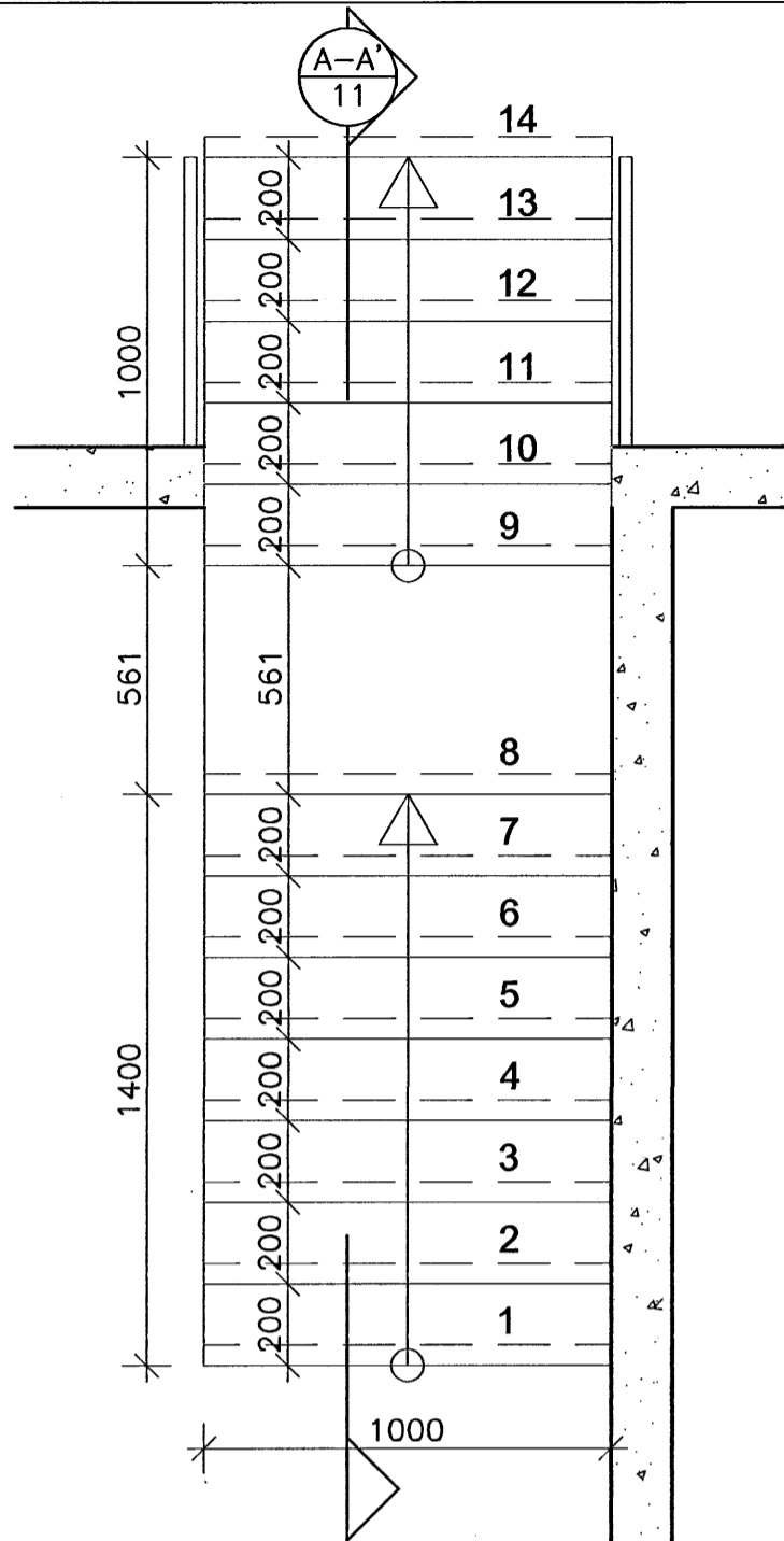
GRUNNMYND STIGA 1, 1:20
