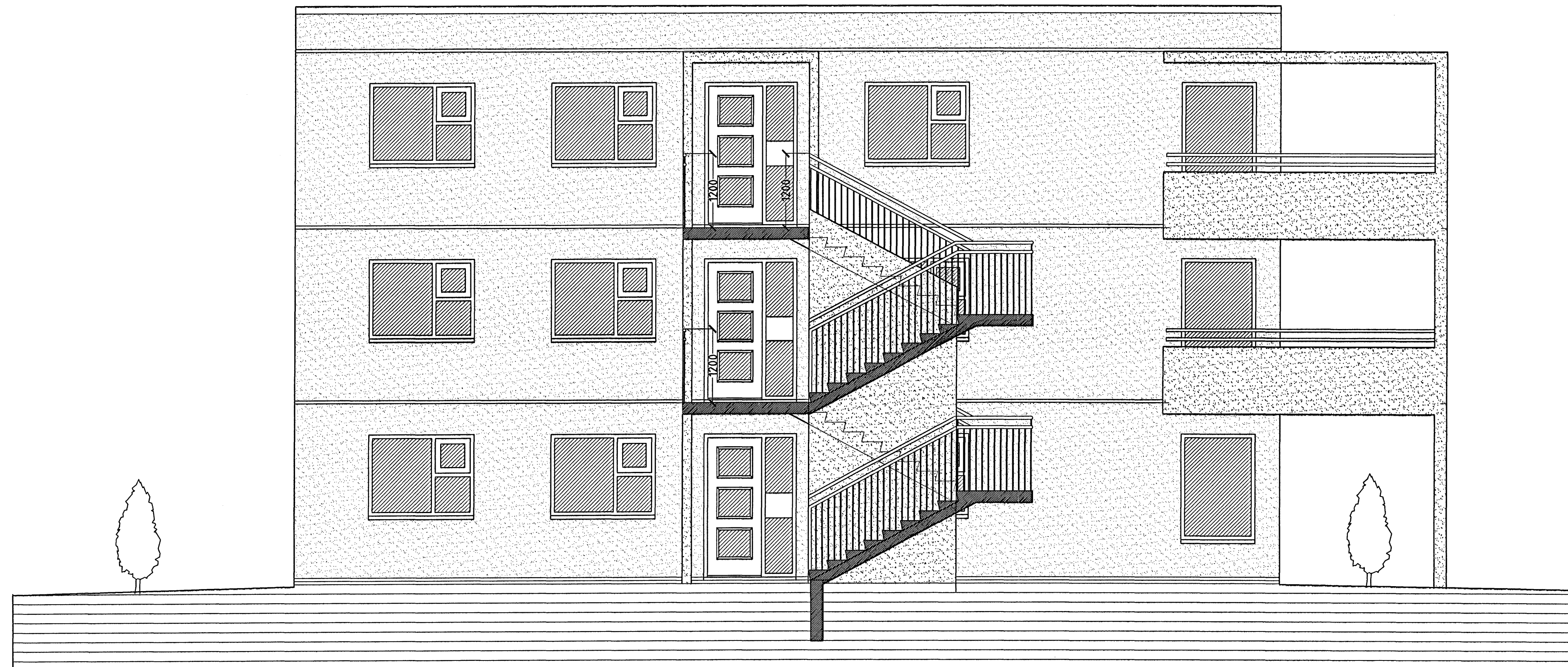
SNID D-D MKV. 1:100.
