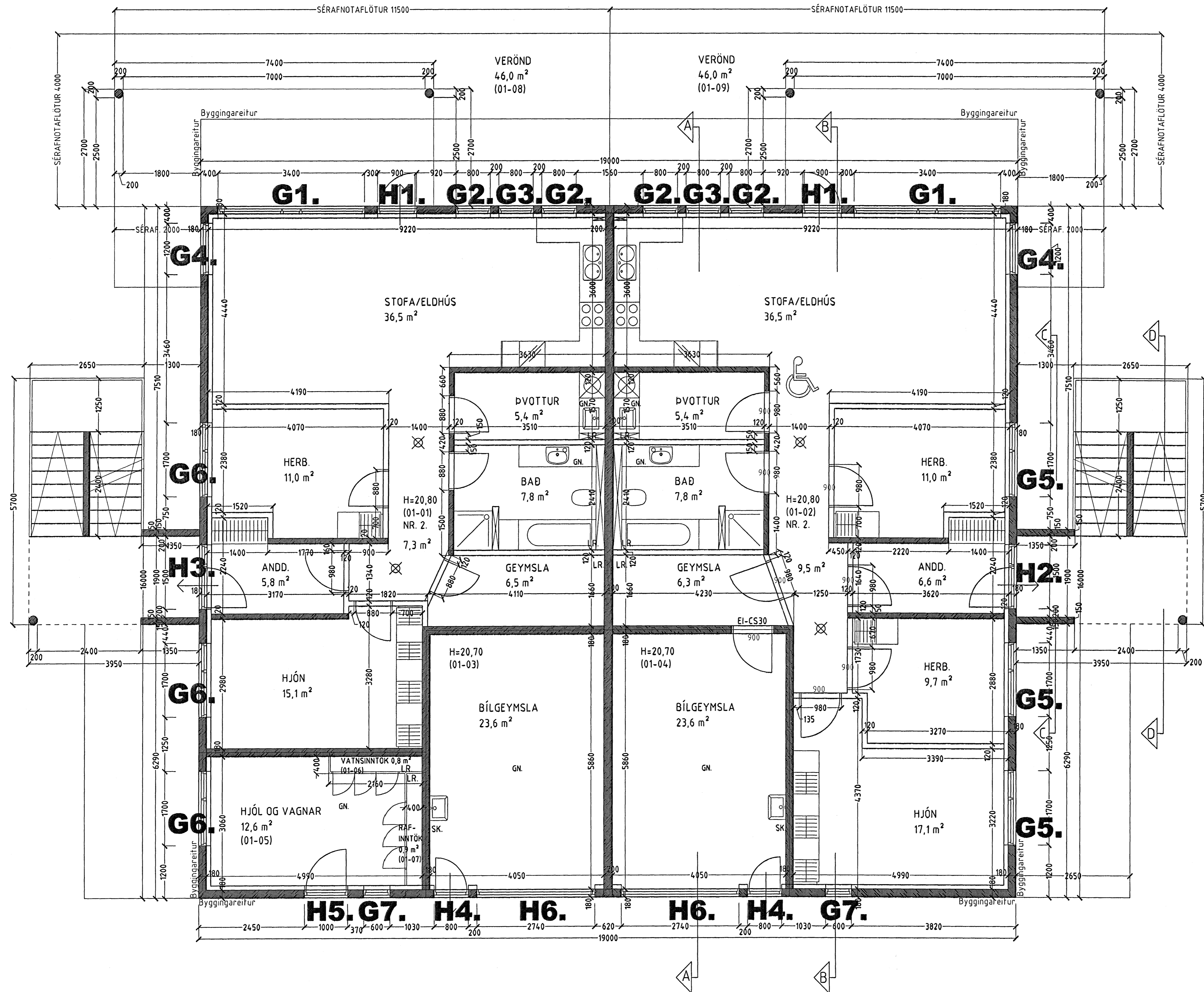
GRUNNMYND 1. HÆÐ MKV. 1:50.
