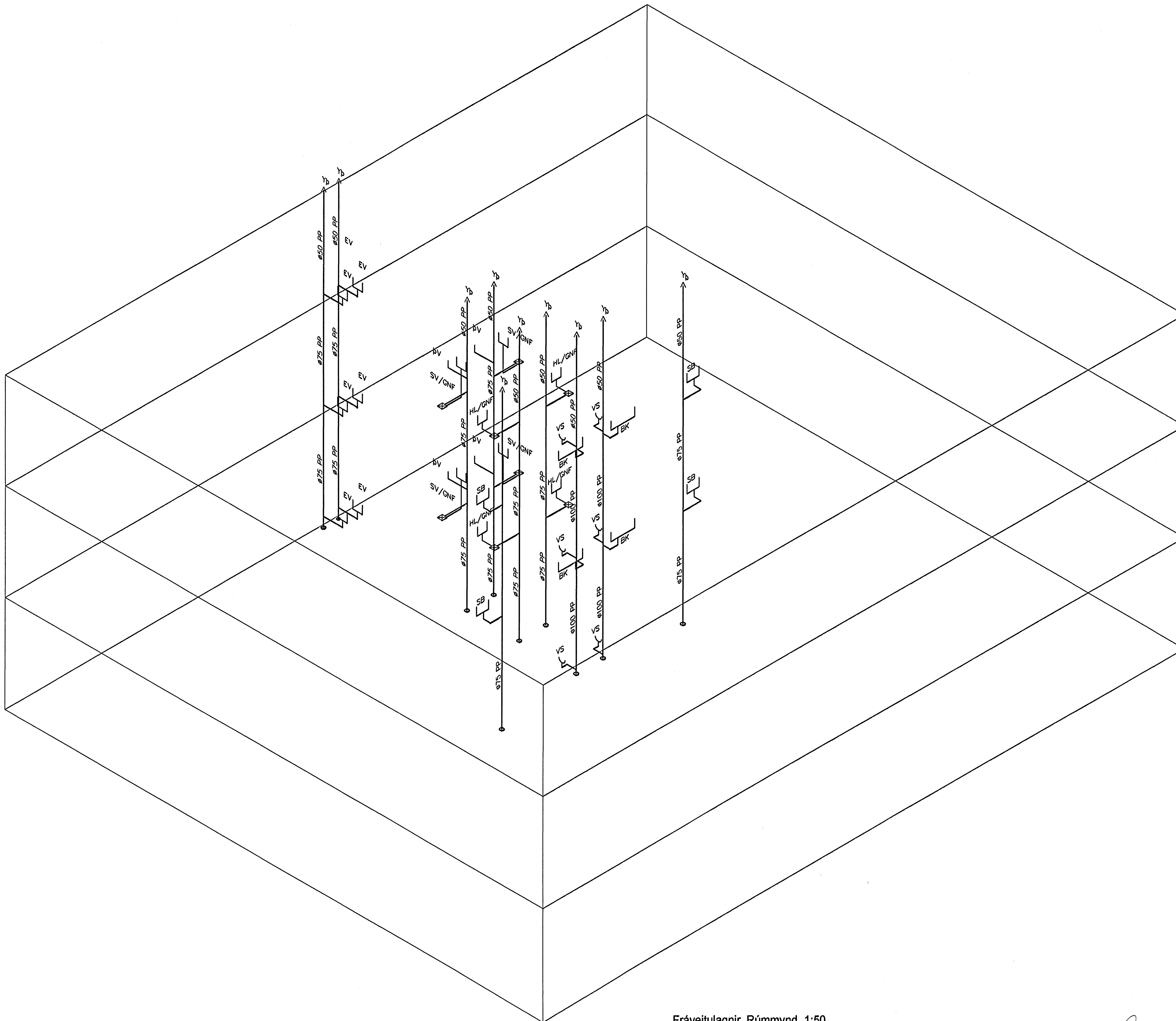
Fráveitulagnir, Rúmmynd, 1:50
