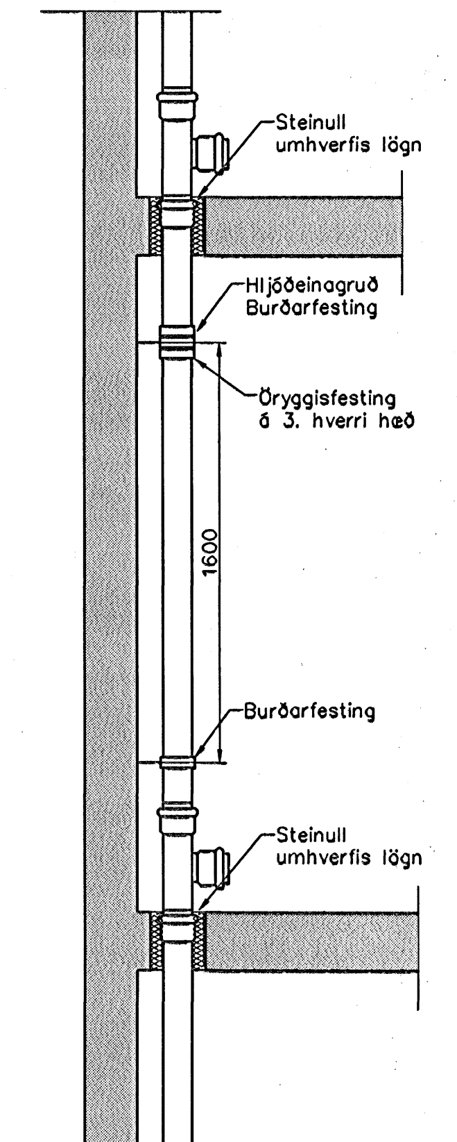
Fallþípa, festingar 1:20
