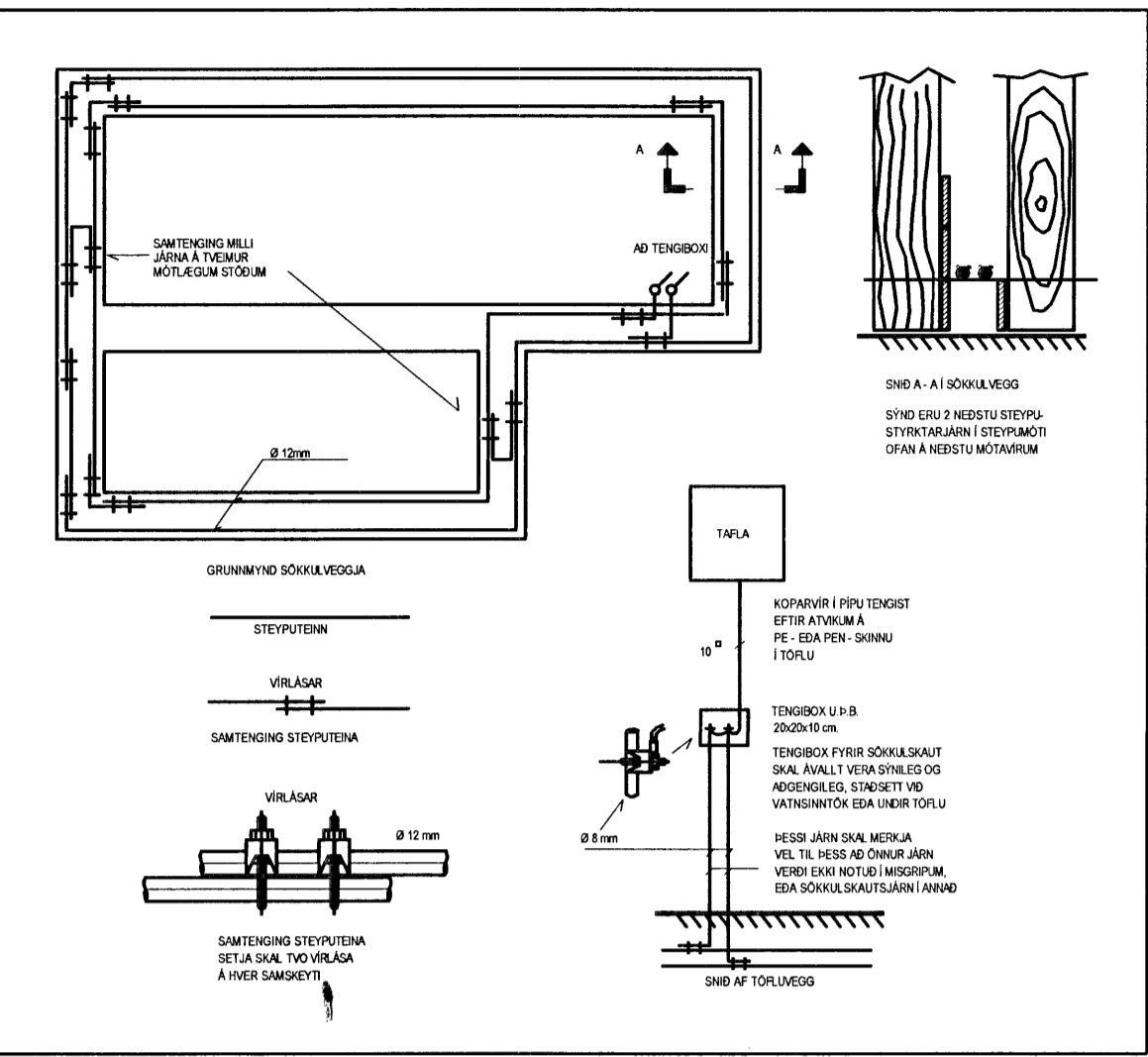
Skýringarmynd sökkulskaut
