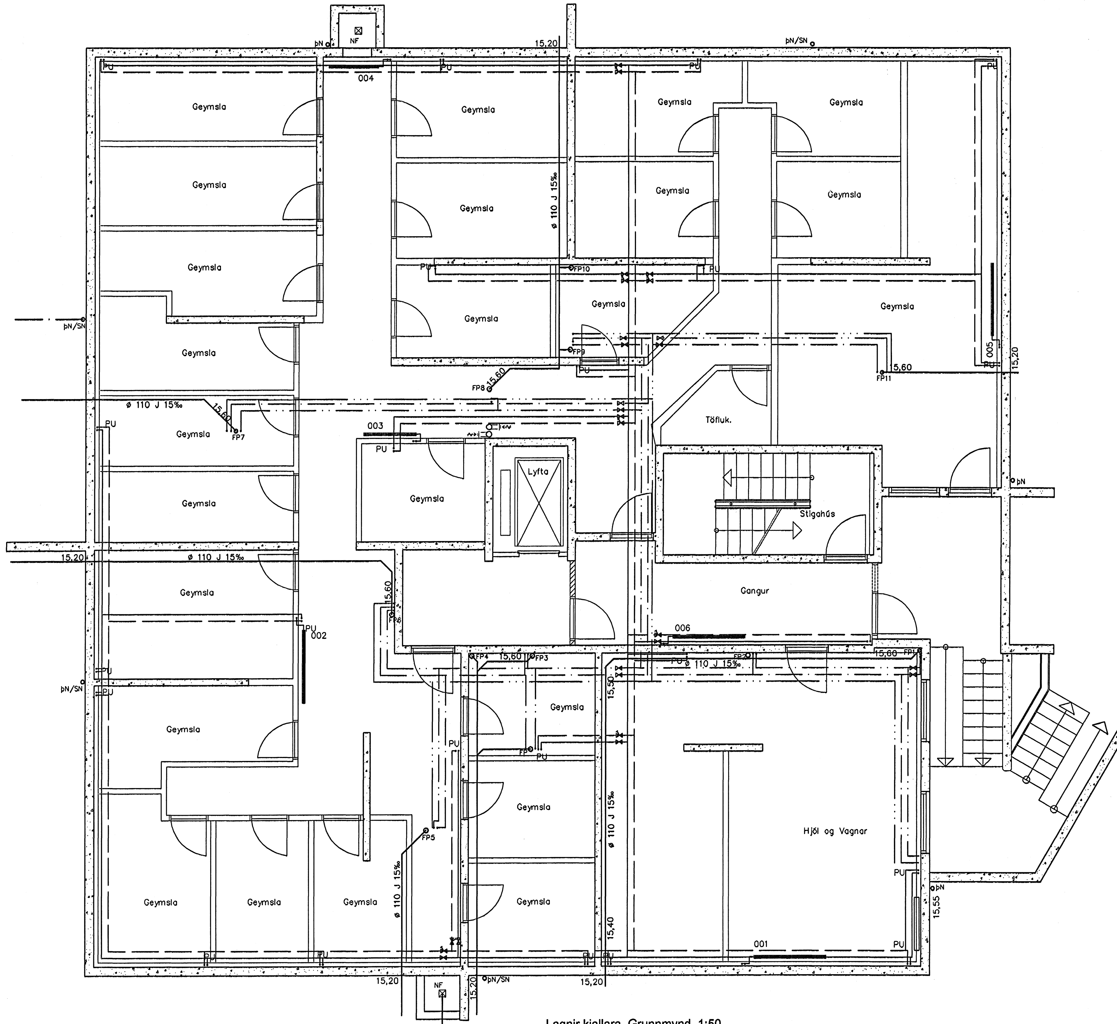
Lagnir kjallara, Grunnmynd, 1:50
