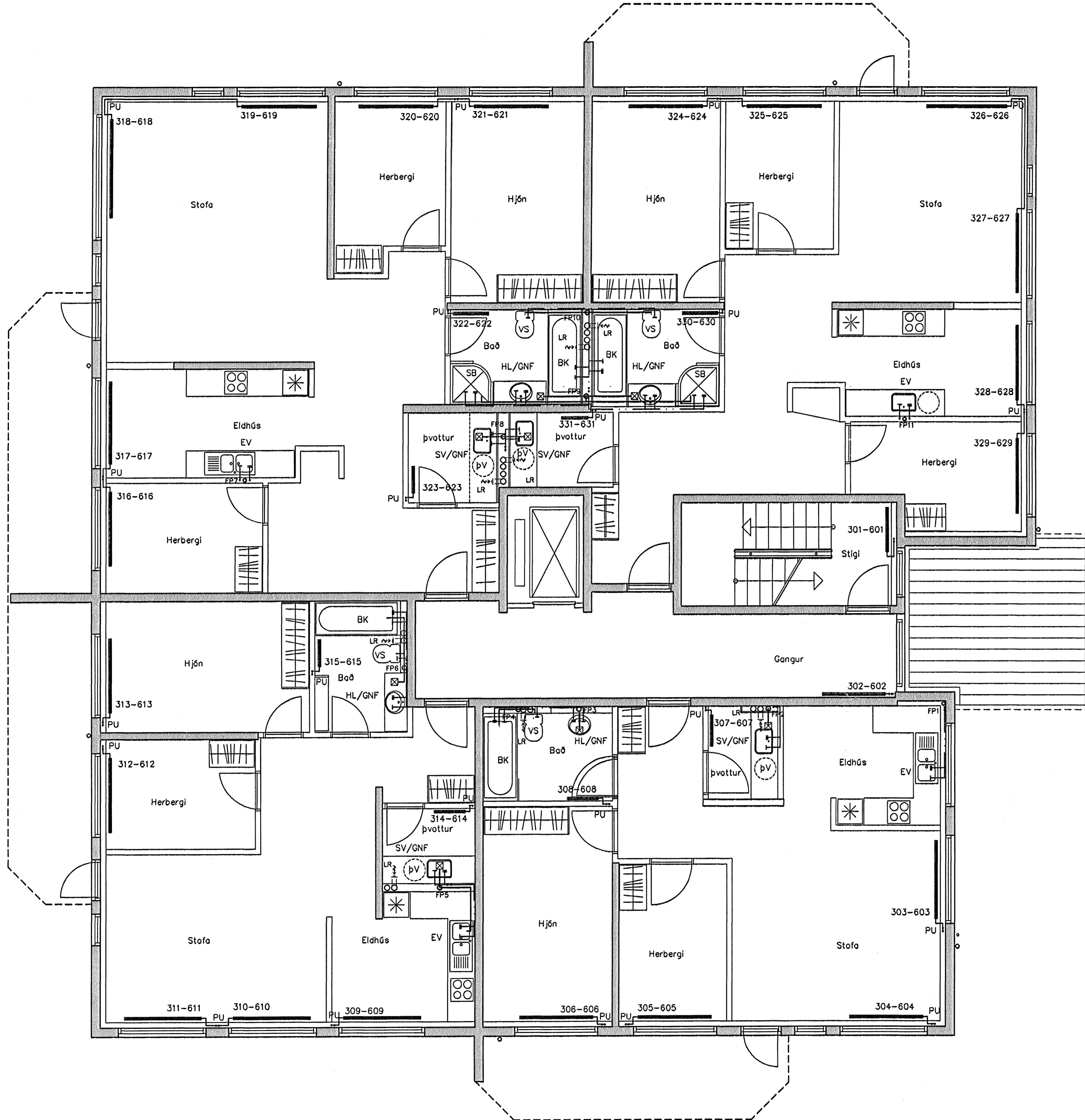
Lagnir 3-6. Hæð, Grunnmynd, 1:50
