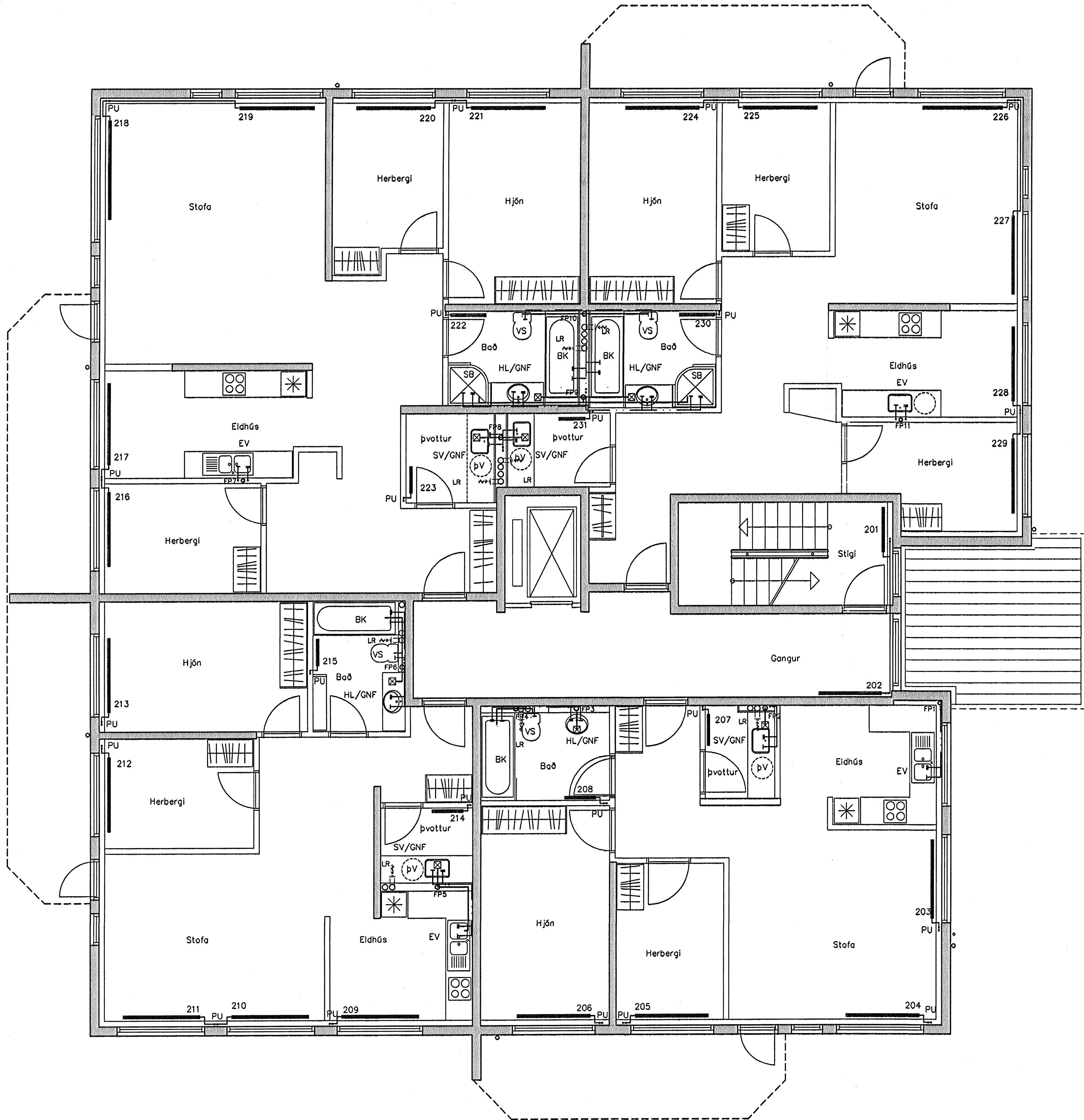
Lagnir 2. Hæð, Grunnmynd, 1:50
