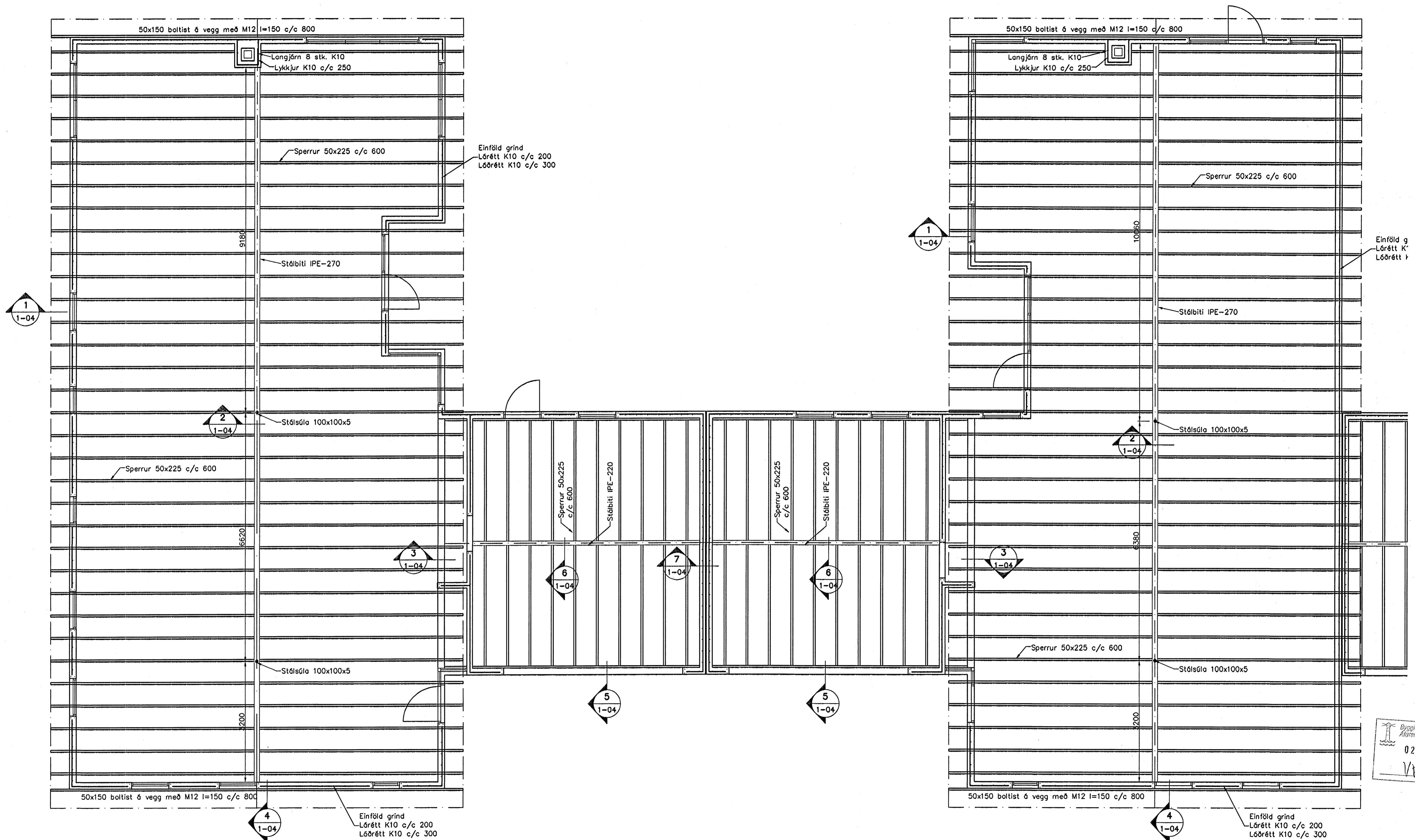
Veggir, þakvirki, Grunnmynd, 1:50
