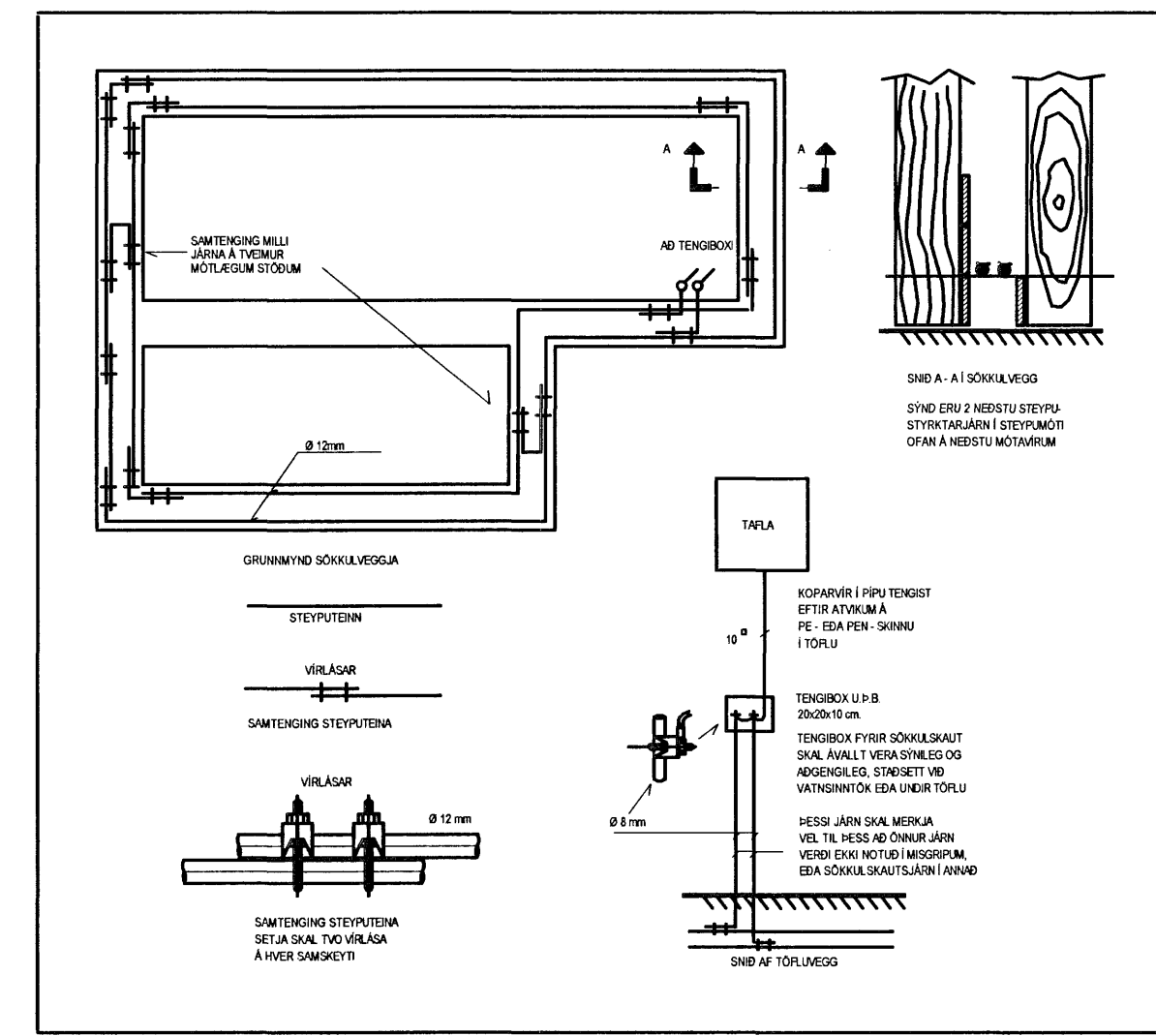
Skýringarmynd sökkulskaut
