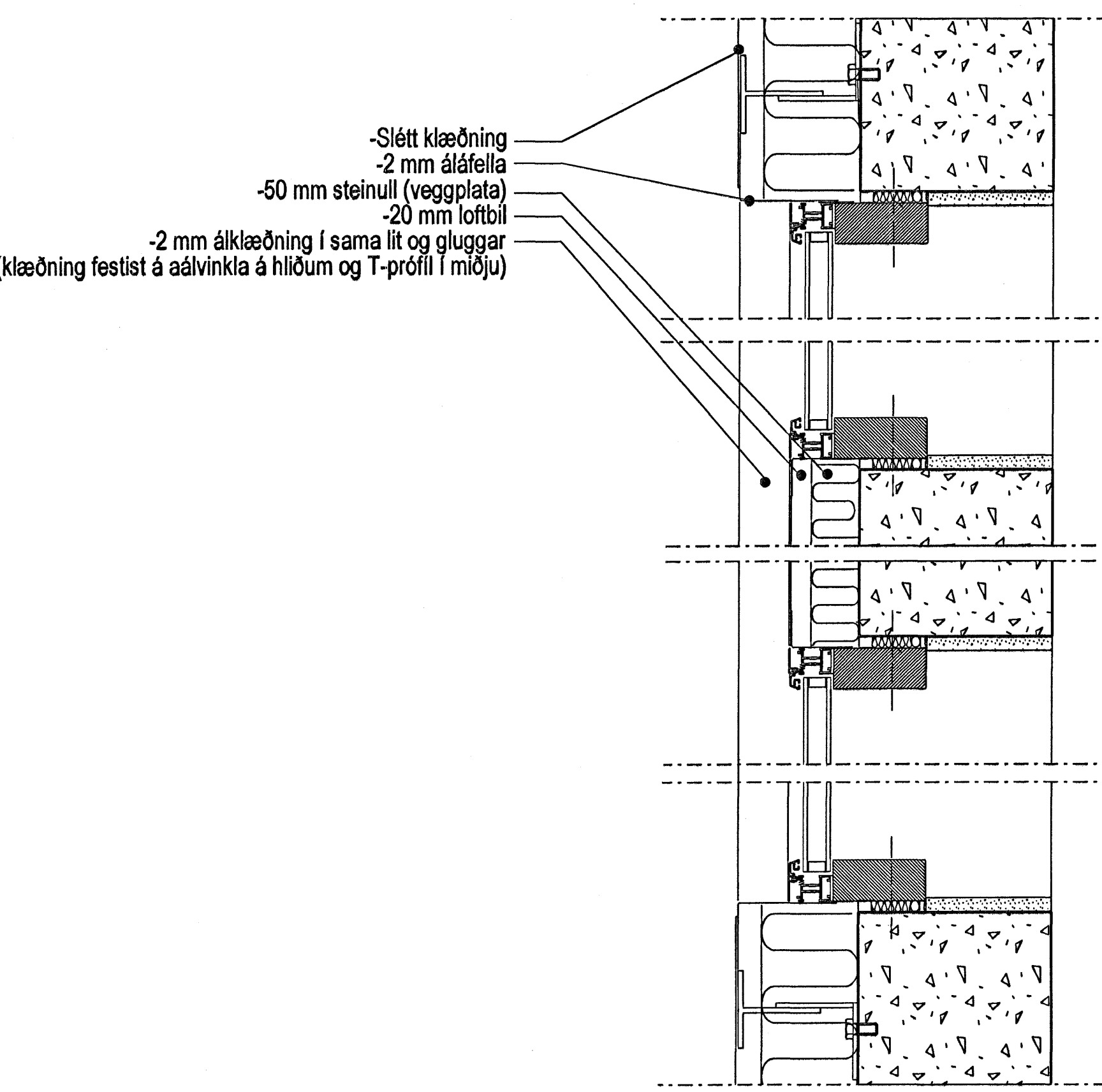
5 - DEILI 1:5 Efri brún gluggaband-báruð álklaðning (líórétt deili)
