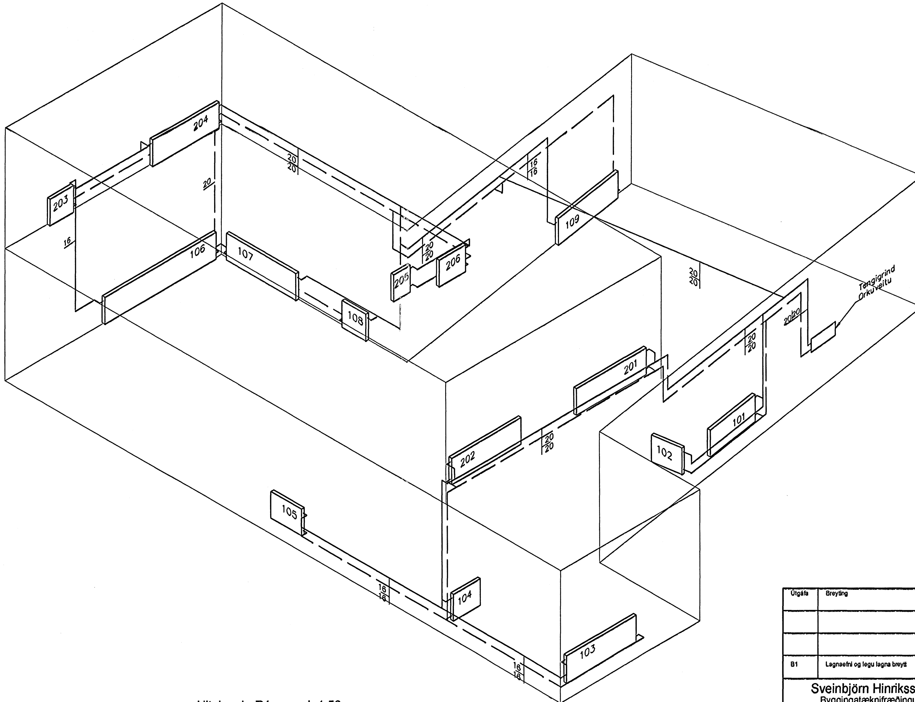
Hitalagnir, Rúmmynd, 1:50
