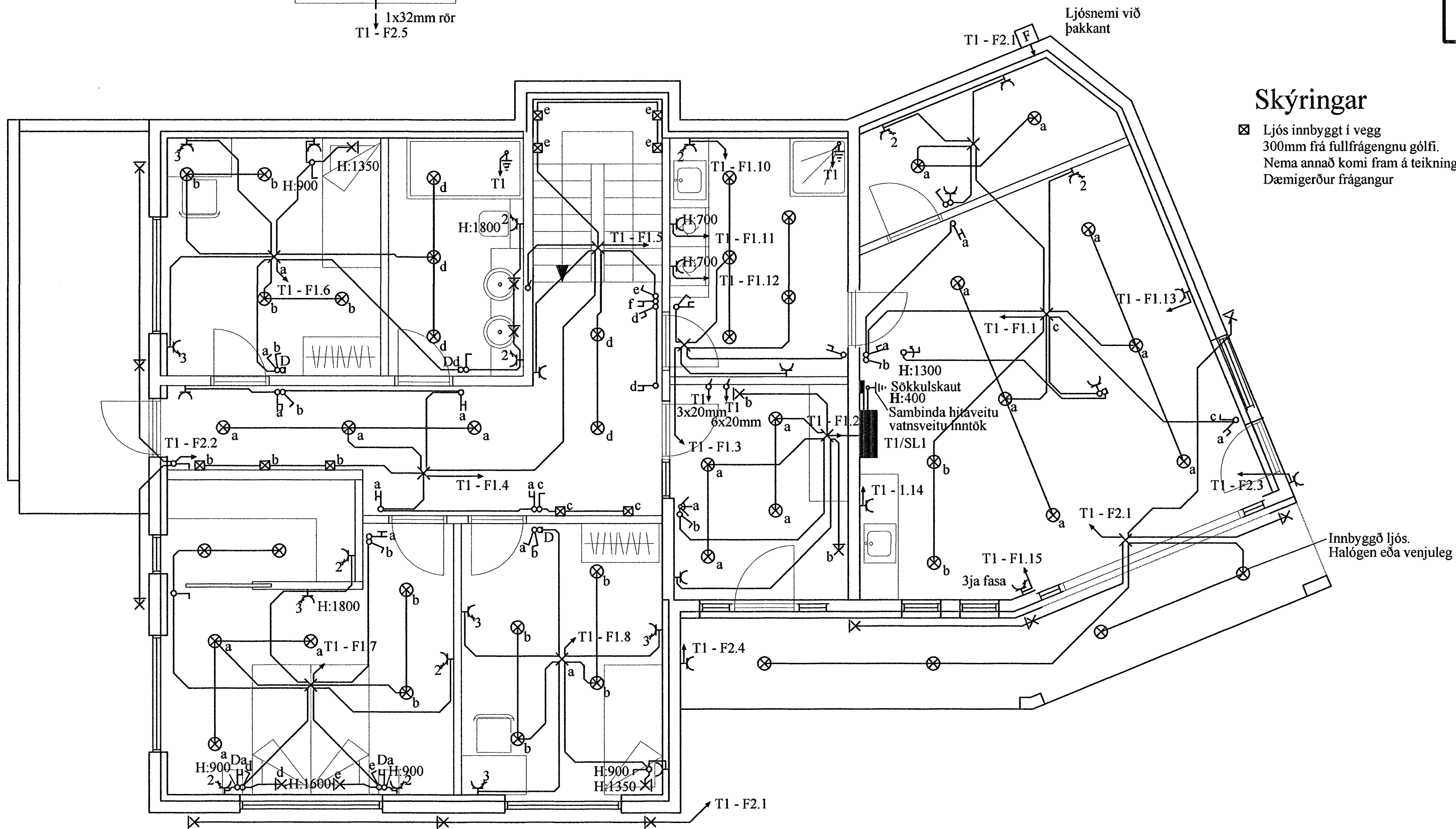
Grunnmynd - Raflögn neðri hæðar
